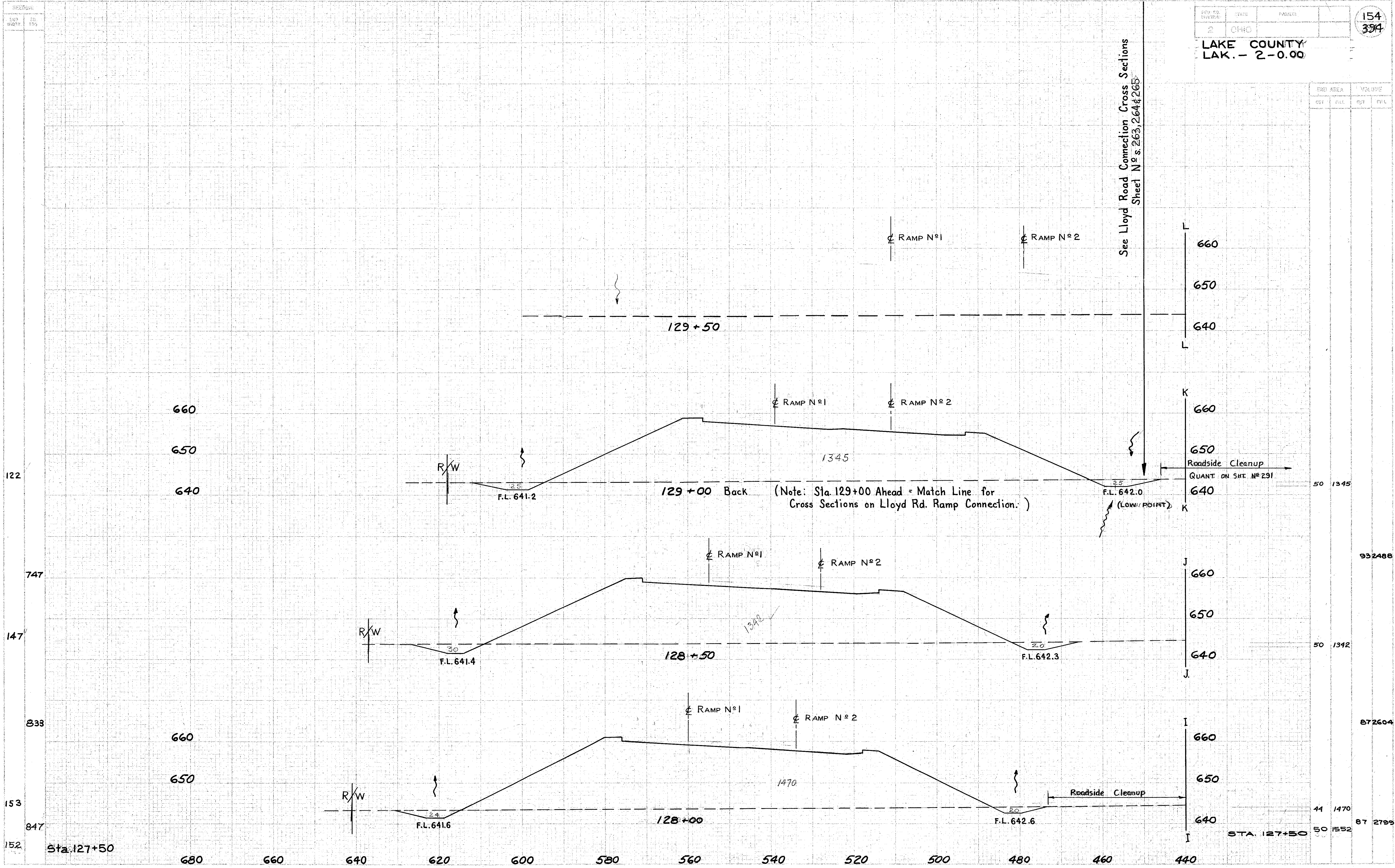
CROSS SECTION EXTENSIONS - STA. 128+00 TO STA. 129+50 - LEFT
