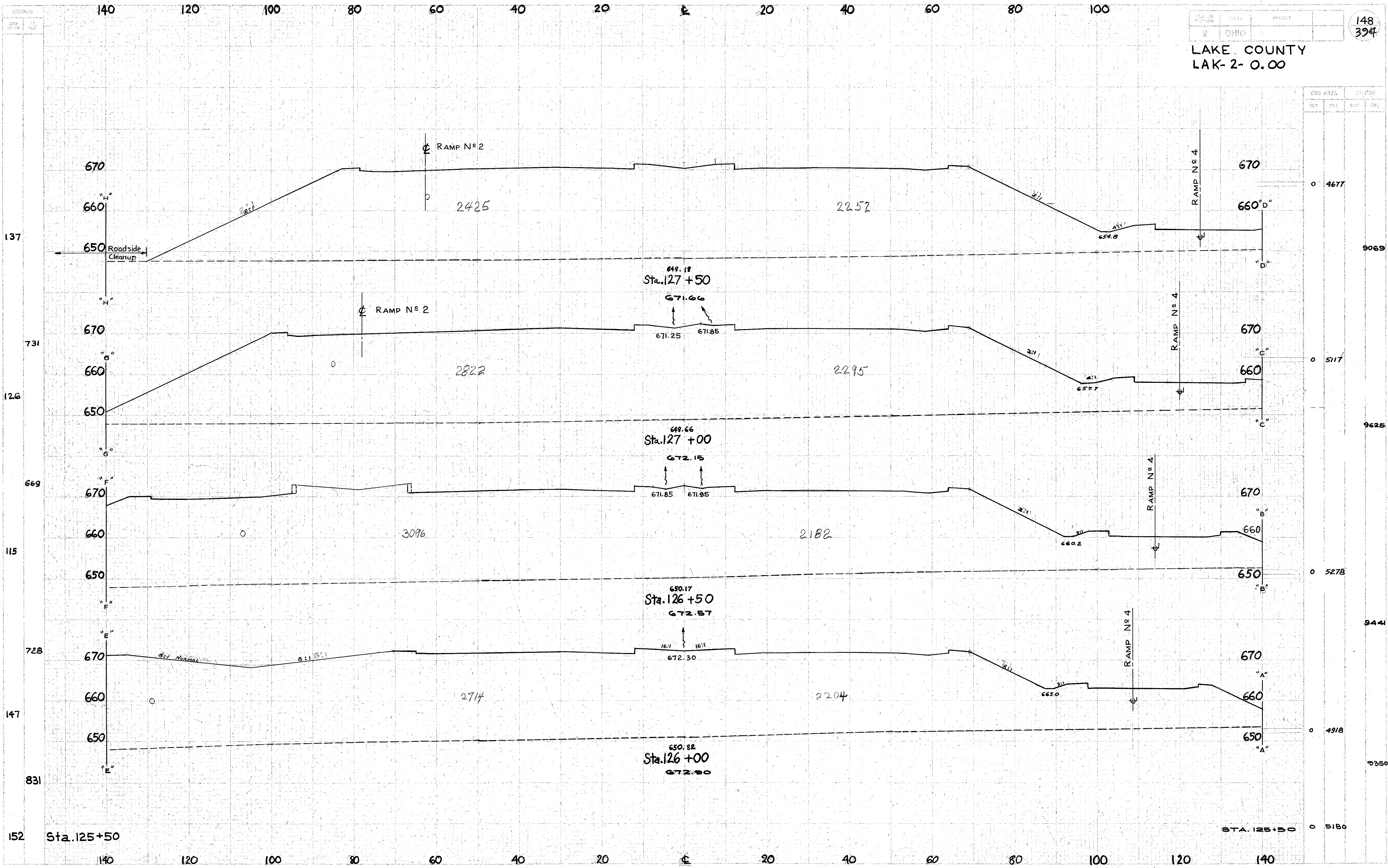
CROSS SECTIONS - STA. 126+00 TO STA. 127+50
