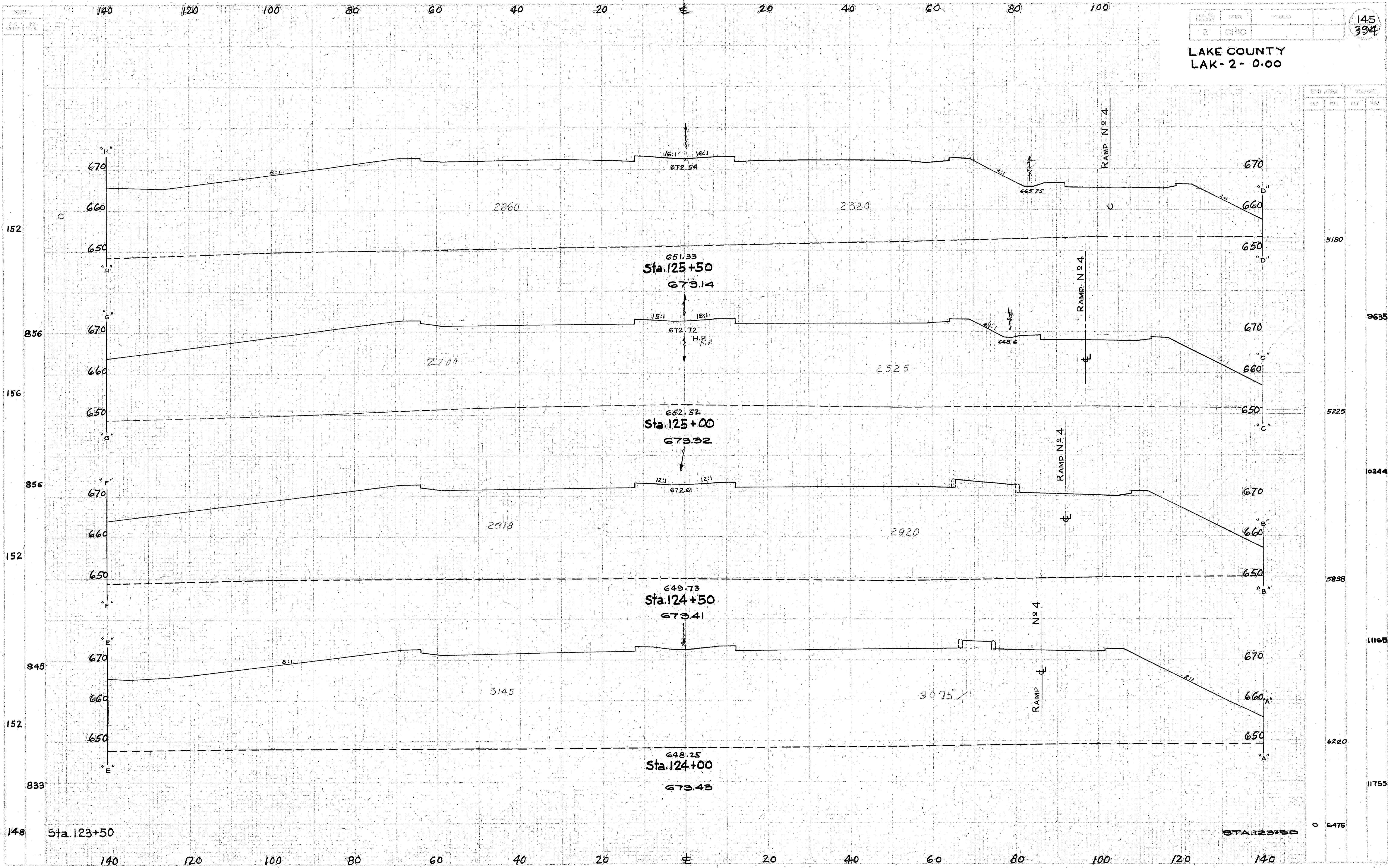
CROSS SECTIONS - STA. 124+00 TO STA. 125+50
