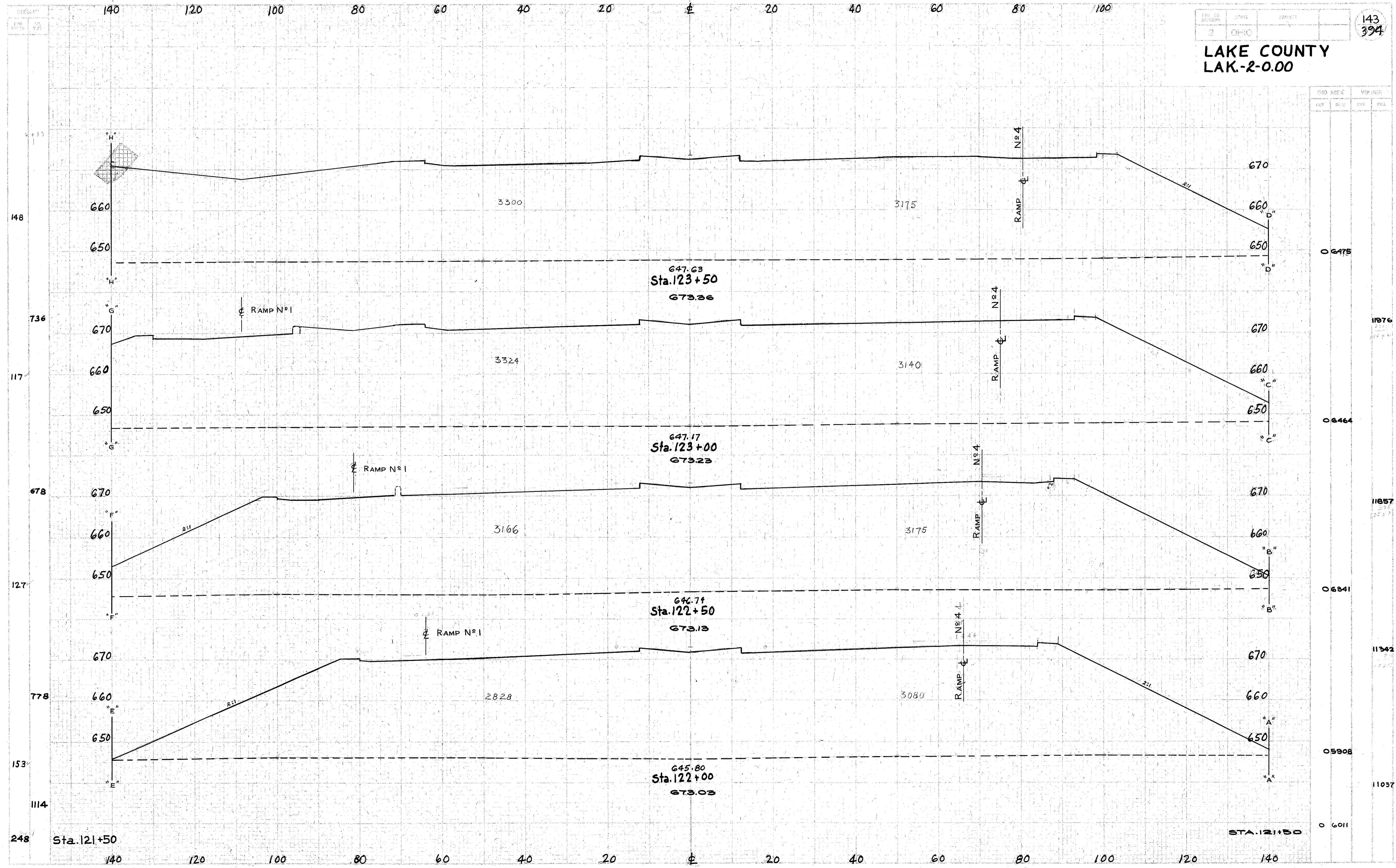
CROSS-SECTIONS - STA. 122+00 TO STA. 123+50
