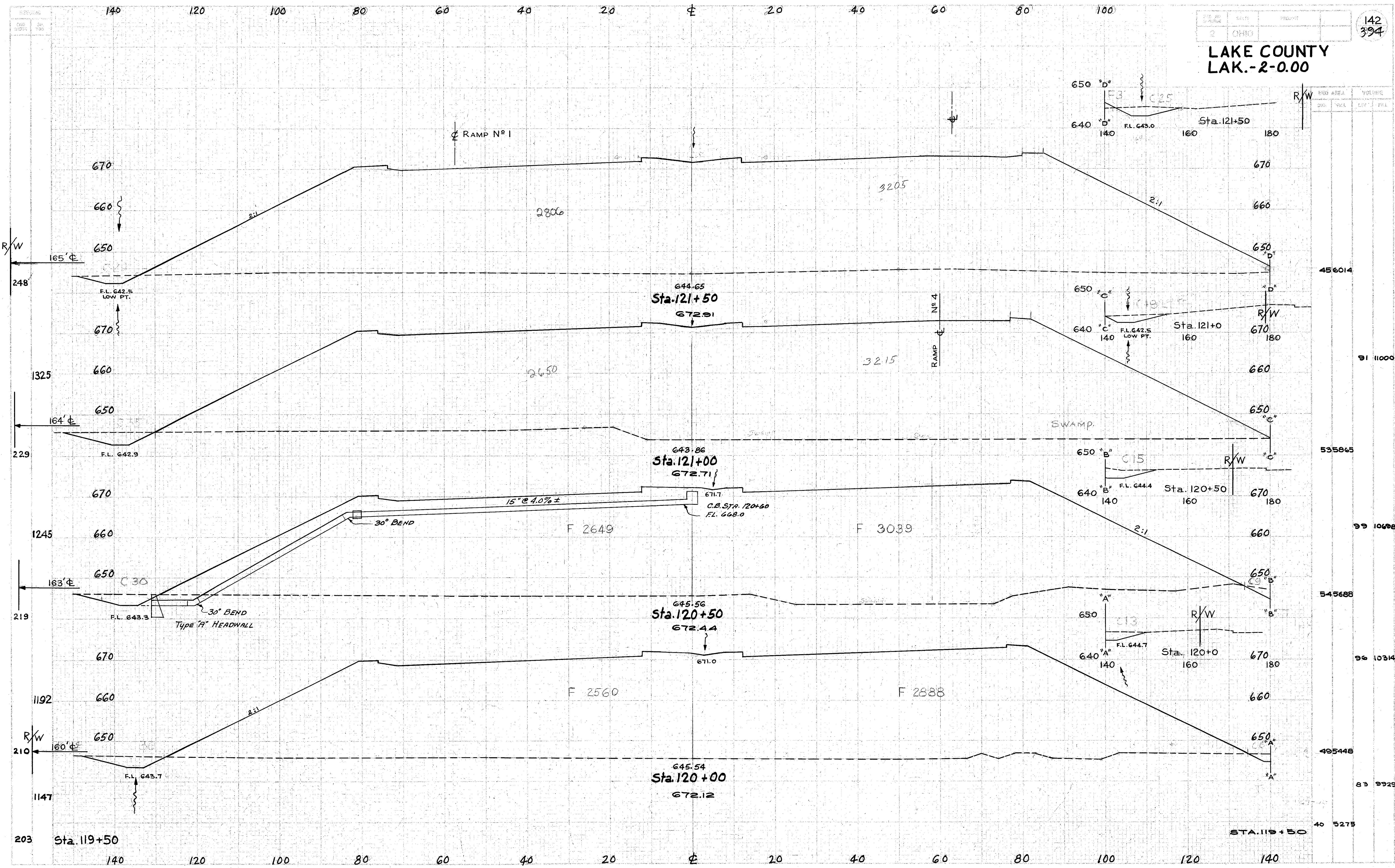
CROSS SECTIONS - STA. 120+00 TO STA. 121+50
