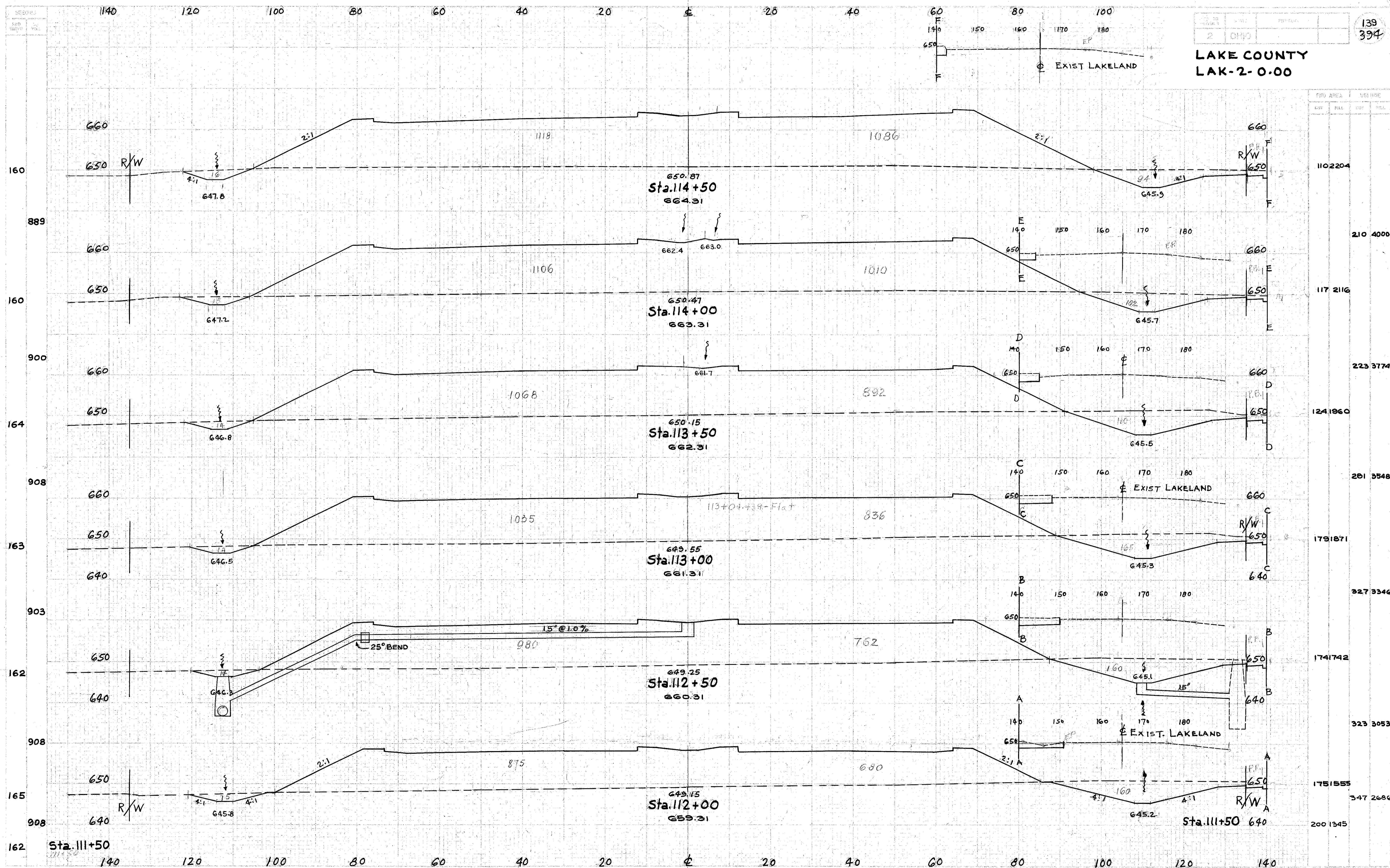
CROSS SECTIONS - STA. 112+00 TO STA. 114+50
