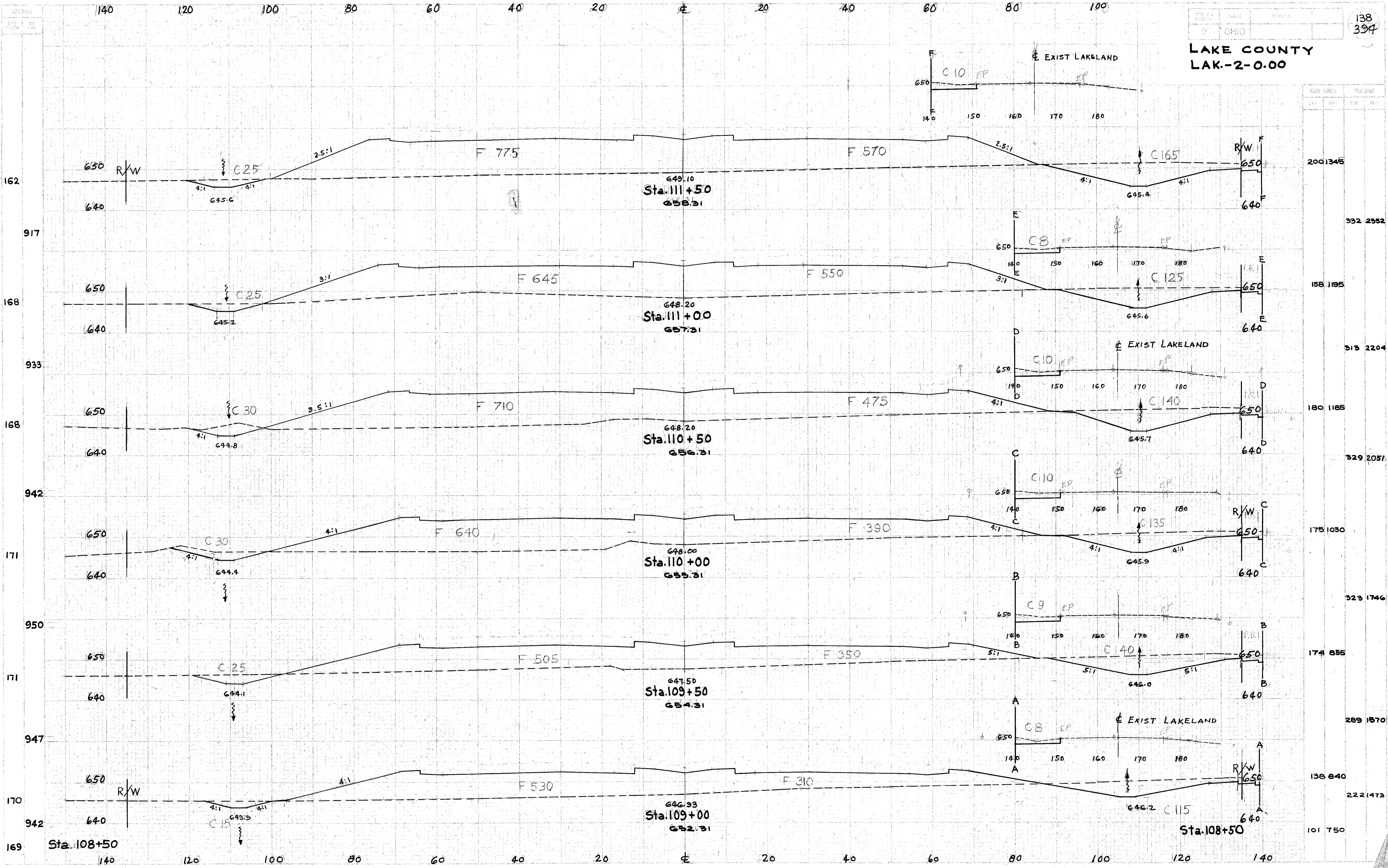
CROSS SECTIONS - STA. 109+00 TO STA. 111+50
