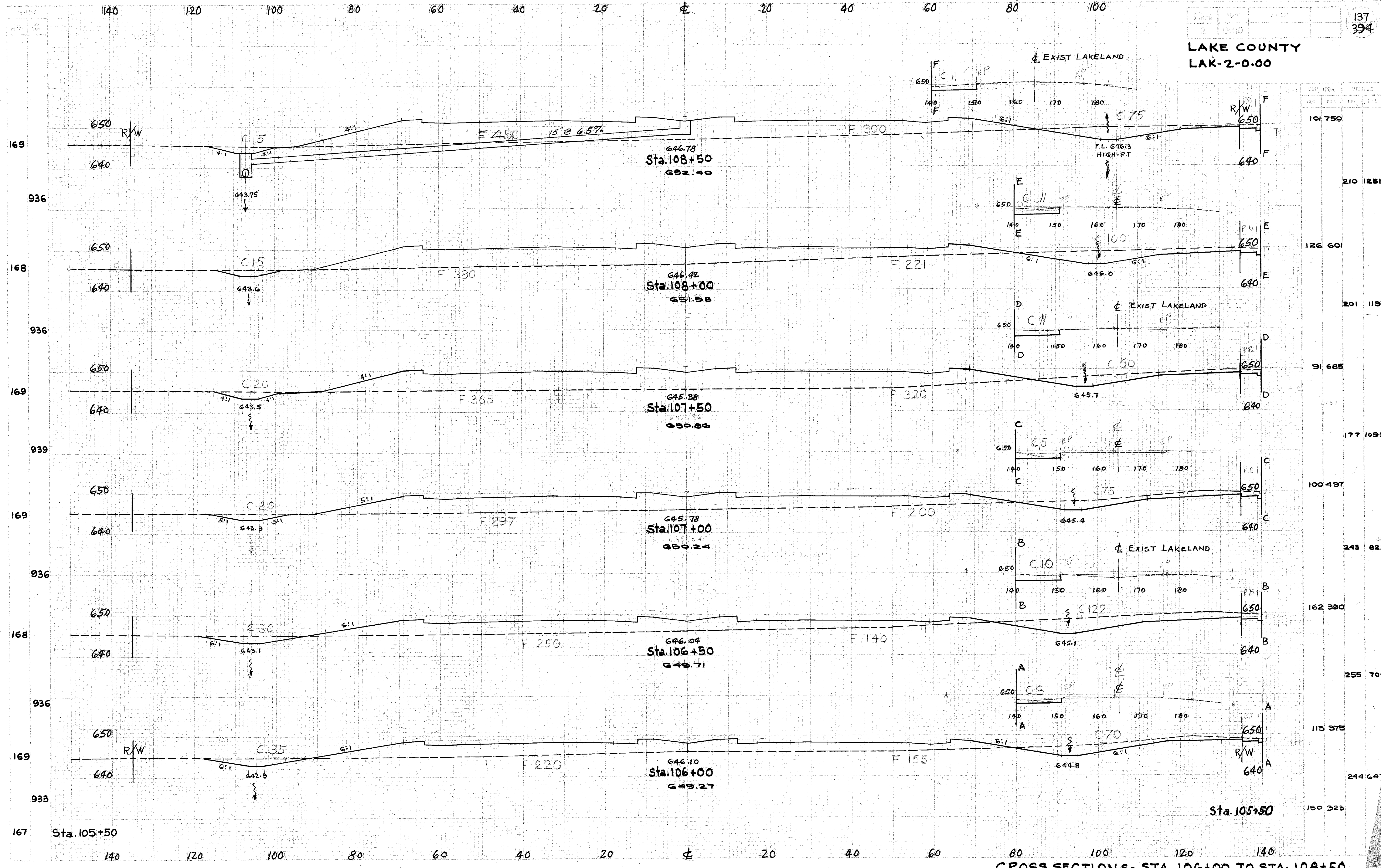
CROSS SECTIONS - STA. 106+00 TO STA. 108+50
