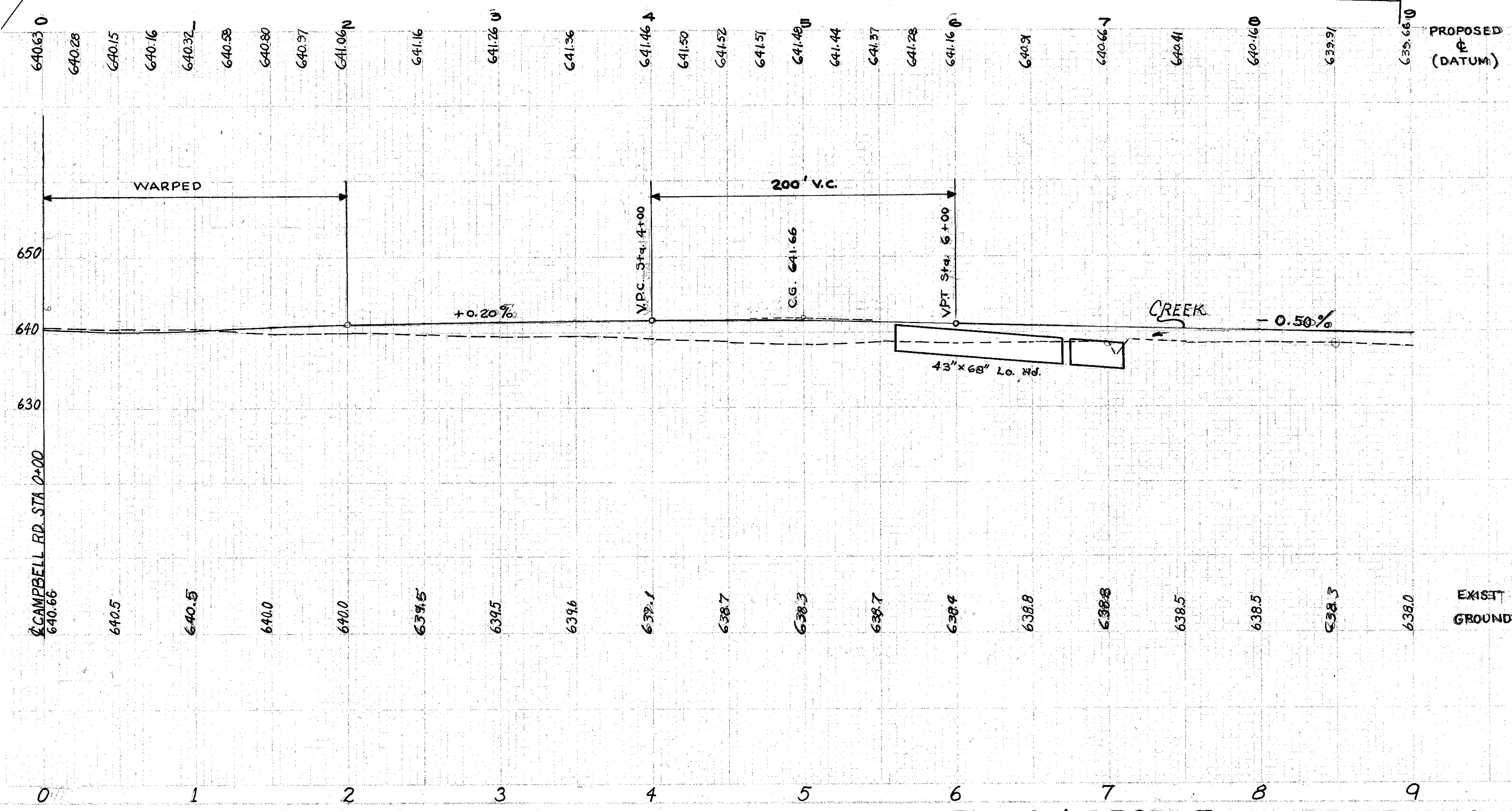
PLAN & PROFILE MARGINAL RD. No 3 STA. 0+00 TO STA. 9+00
