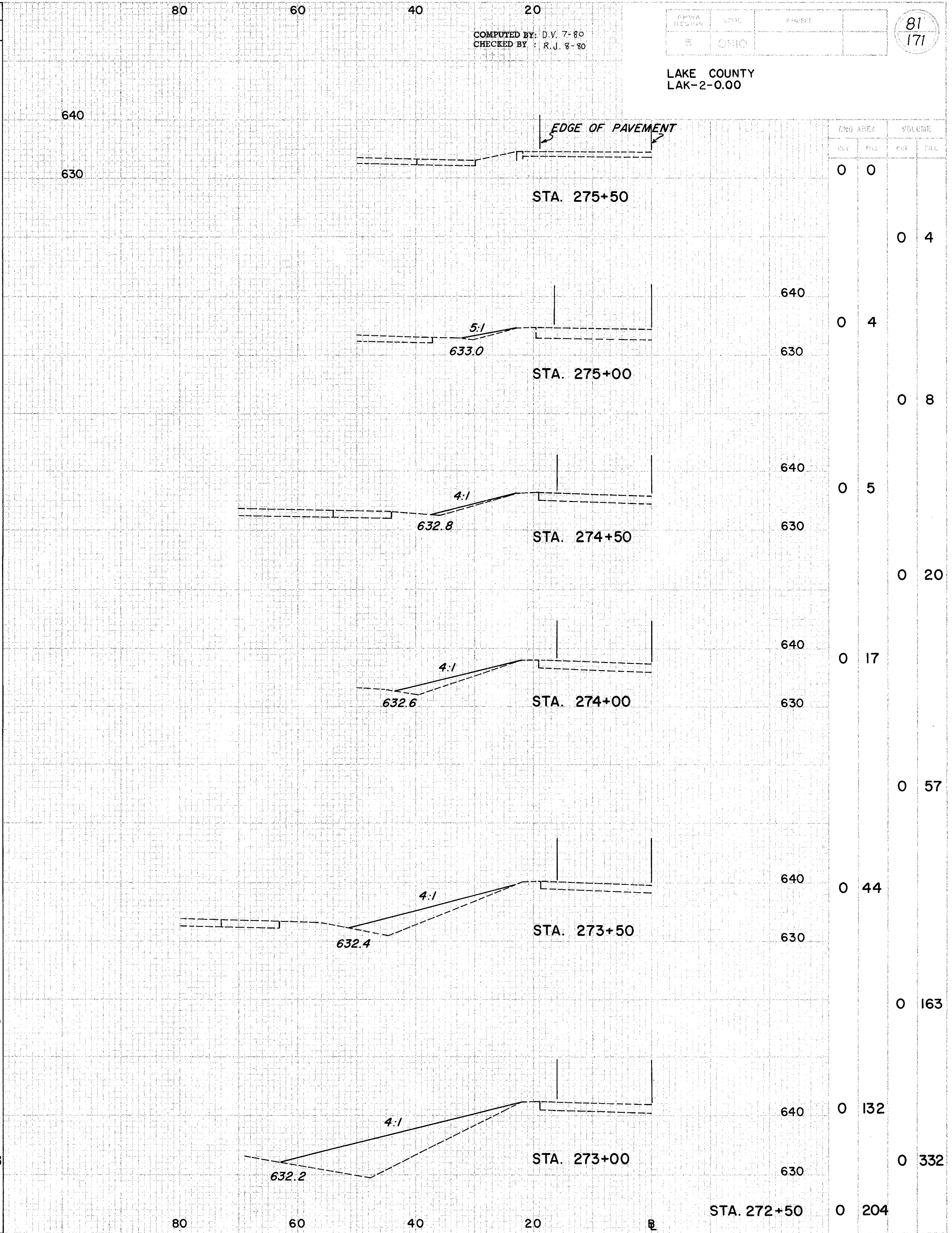
RAMP C-3 STA. 270+50 TO STA. 275+50
