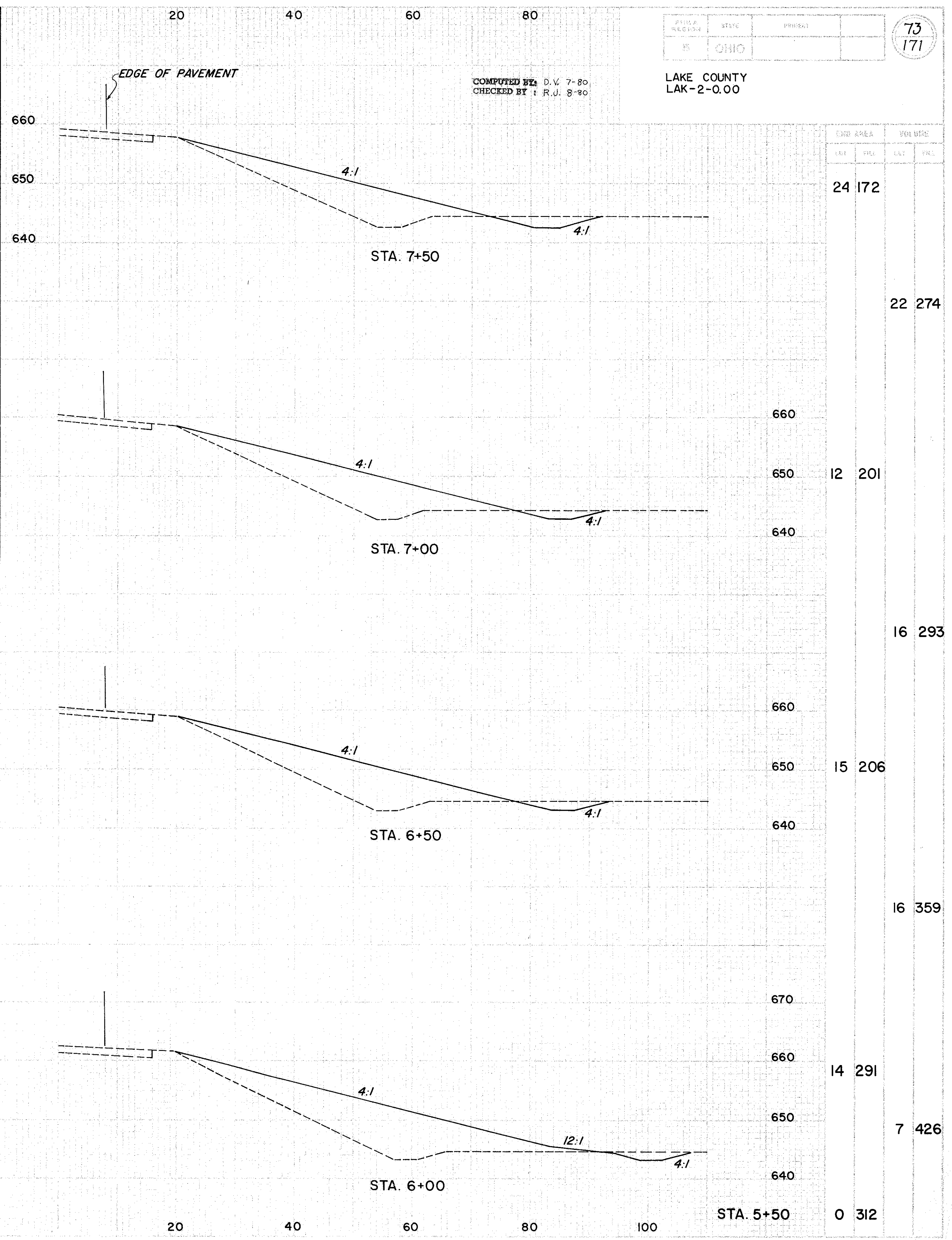
RAMP A-2 STA. 4+00 TO STA. 7+50
