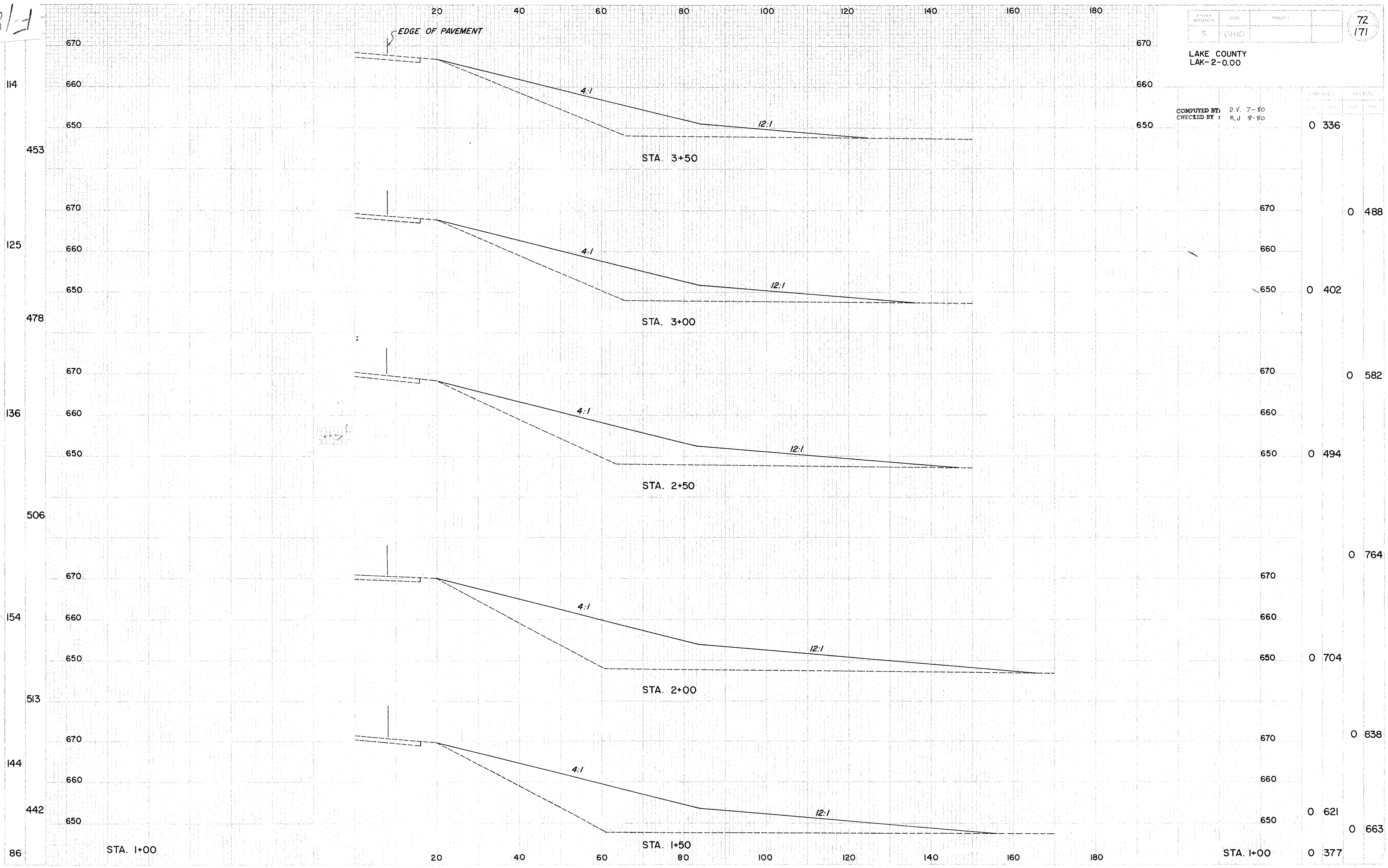
RAMP A-2 STA. 1+50 TO STA. 3+50
