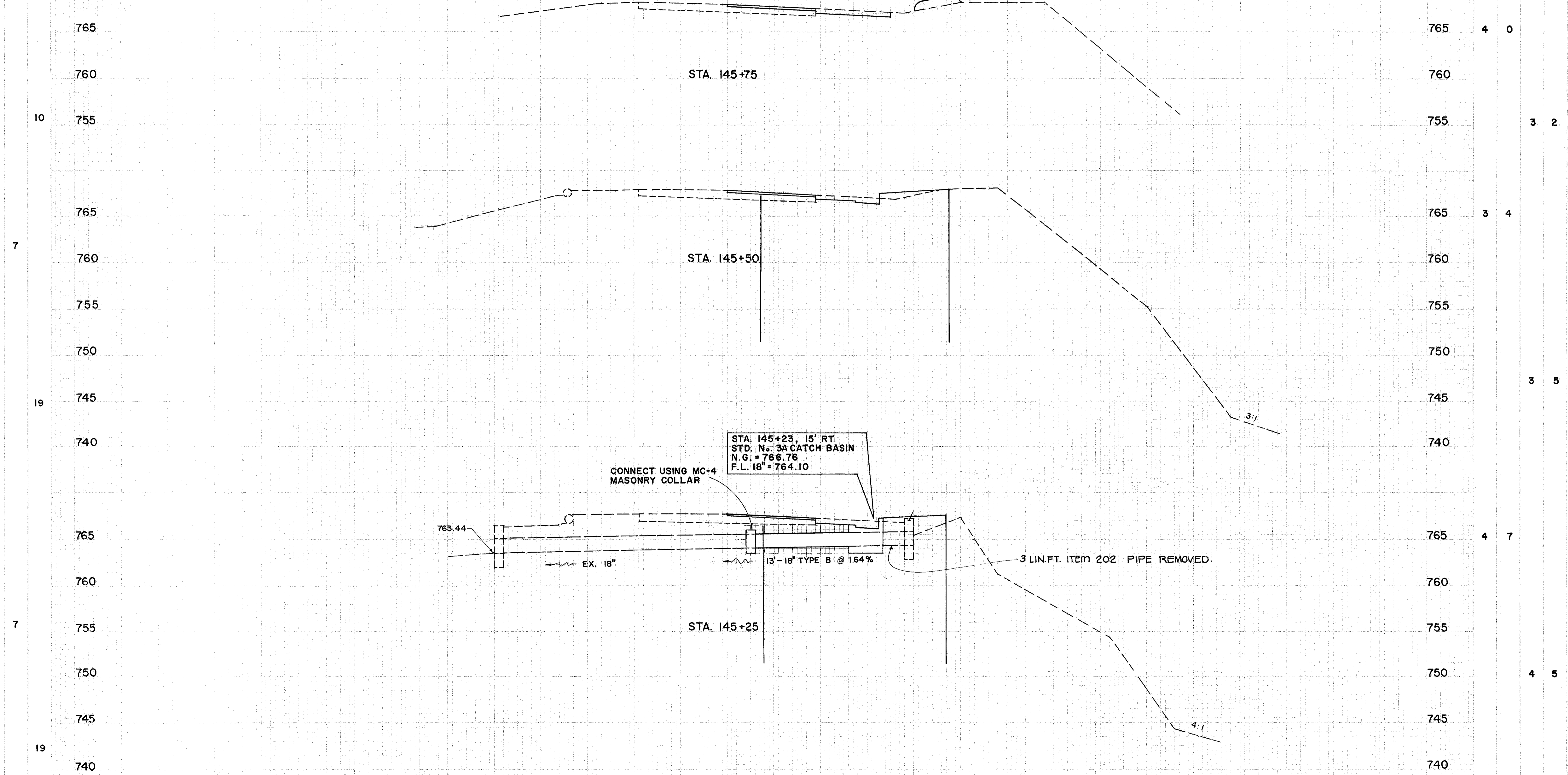
CROSS SECTIONS STA. 145+25 TO STA. 145+75
