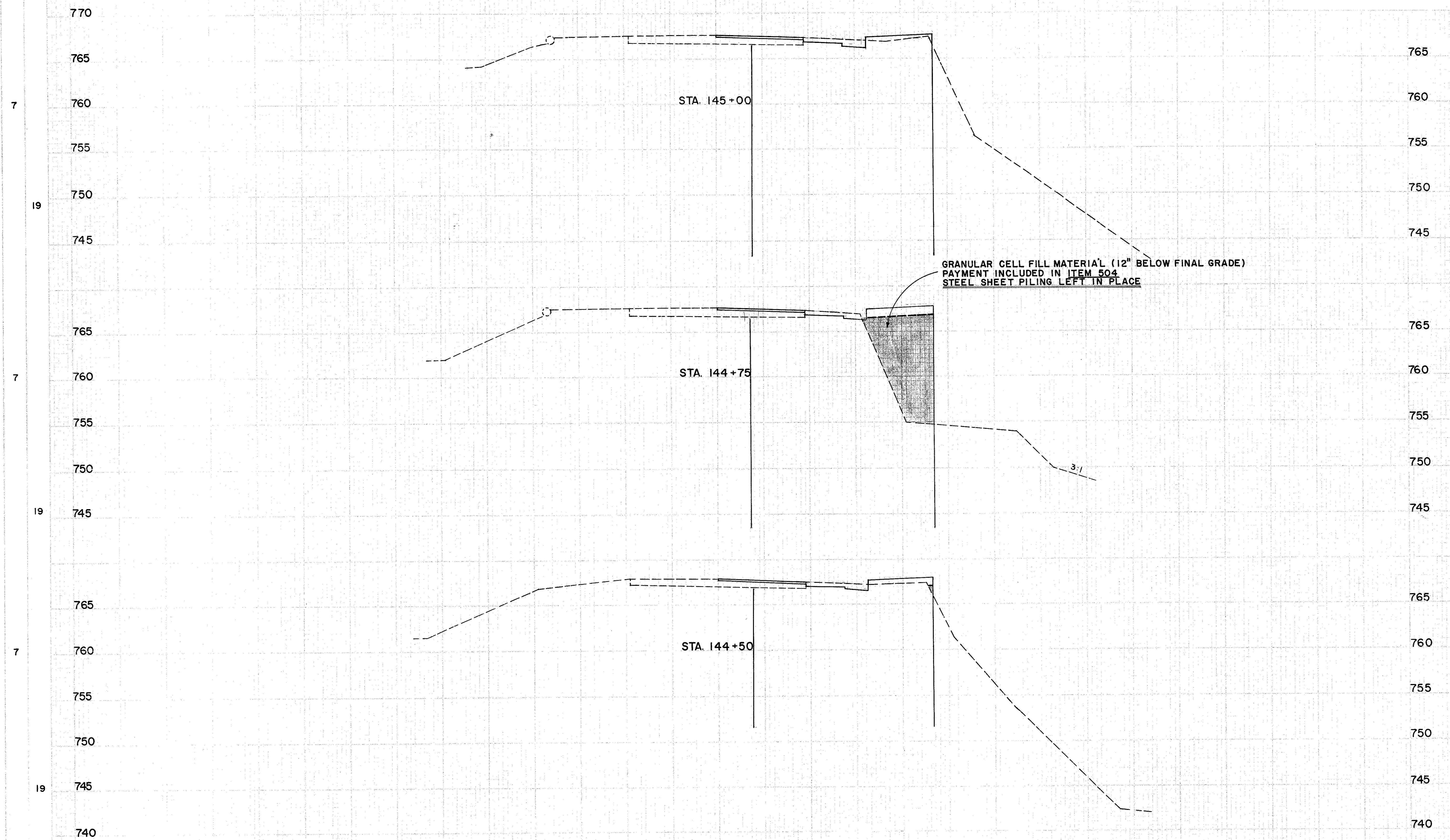
CROSS SECTIONS STA. 144+50 TO STA. 145+00
