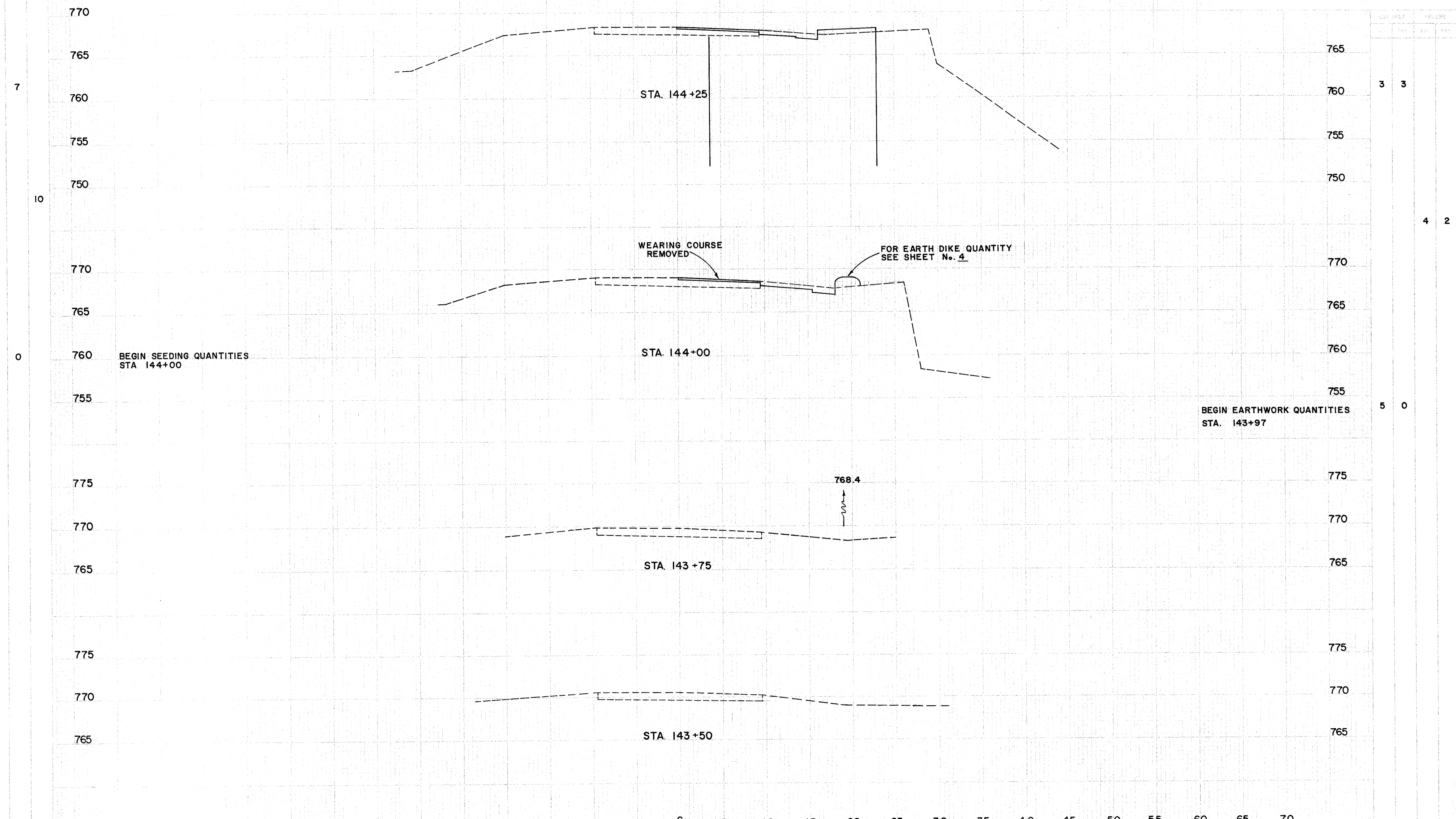
CROSS SECTIONS STA. 143+50 TO STA. 144+25
