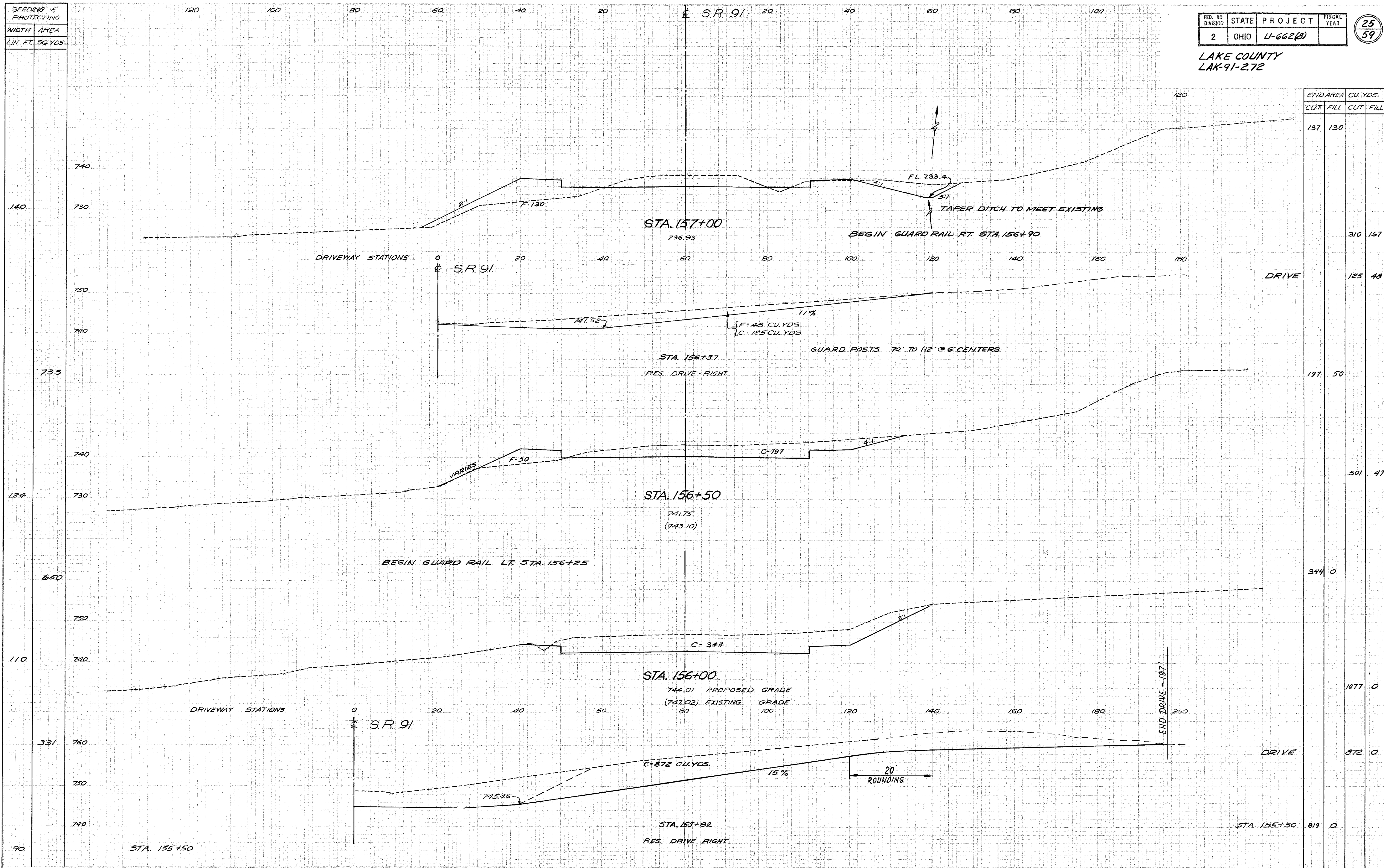
Cross Sections STA. 156+00 To STA. 157+00
