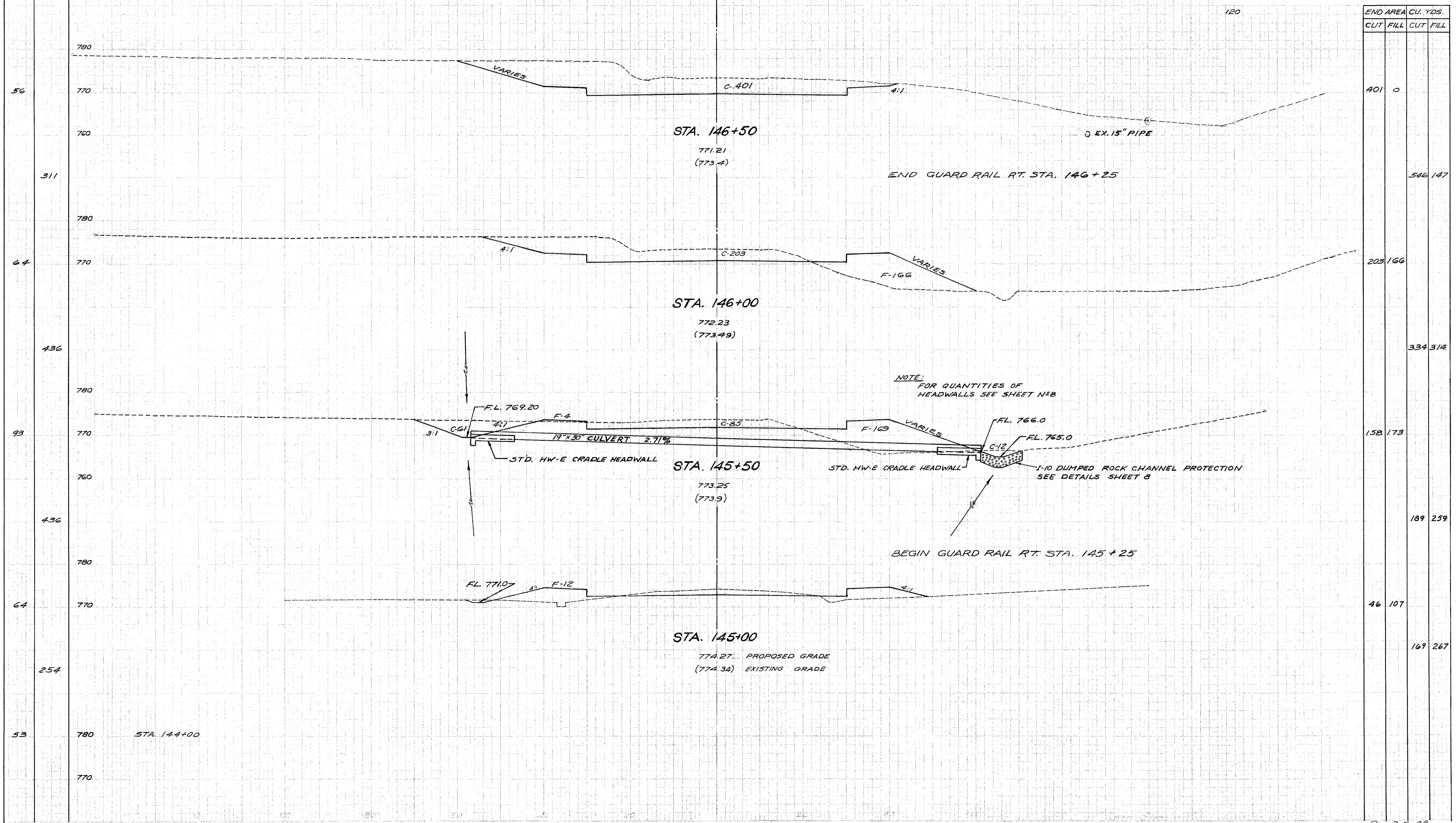
Cross Sections STA. 145+00 To STA. 146+50
