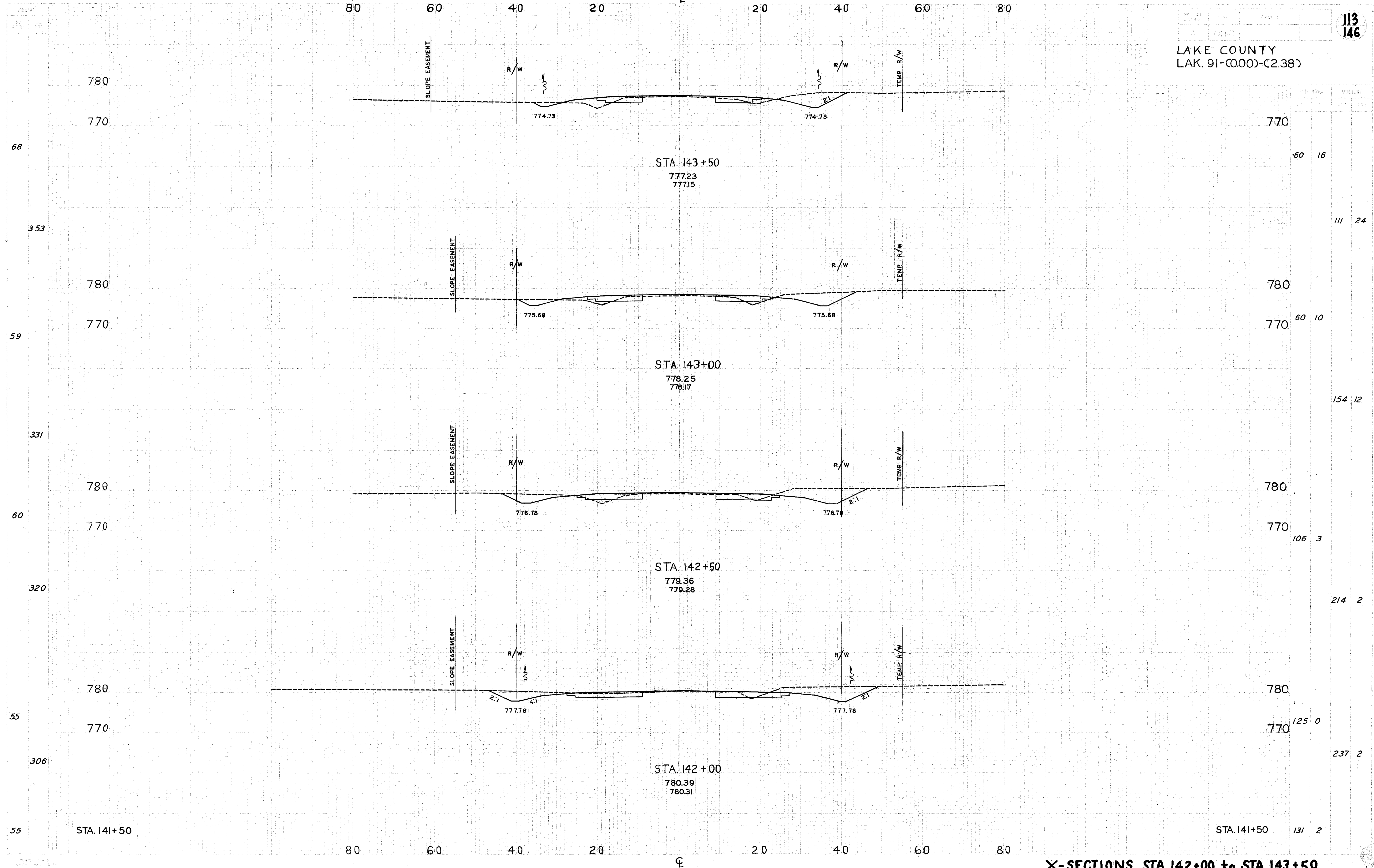
X-SECTIONS STA. 142+00 to STA. 143+50
