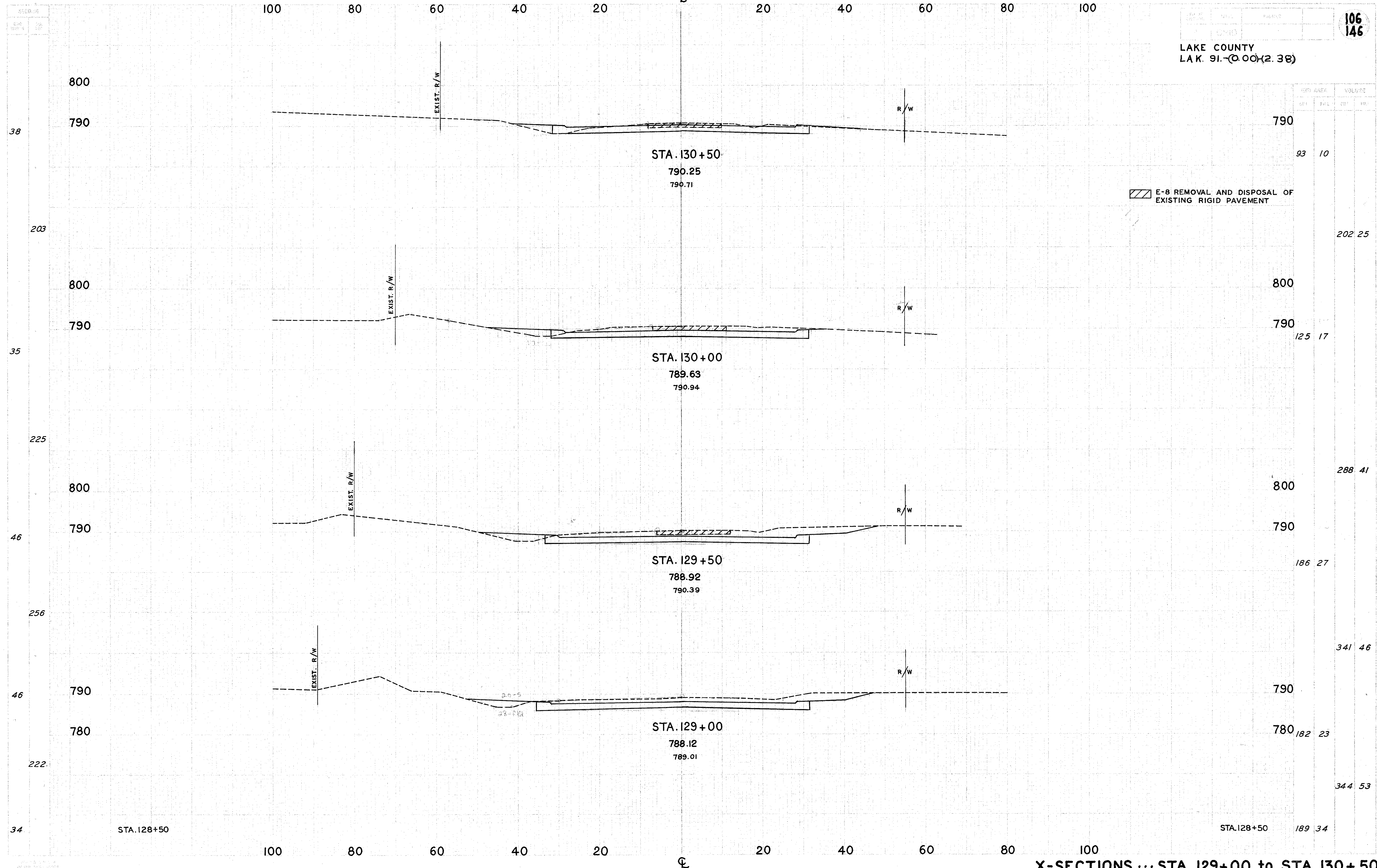
X-SECTIONS ... STA. 129+00 to STA. 130+50
