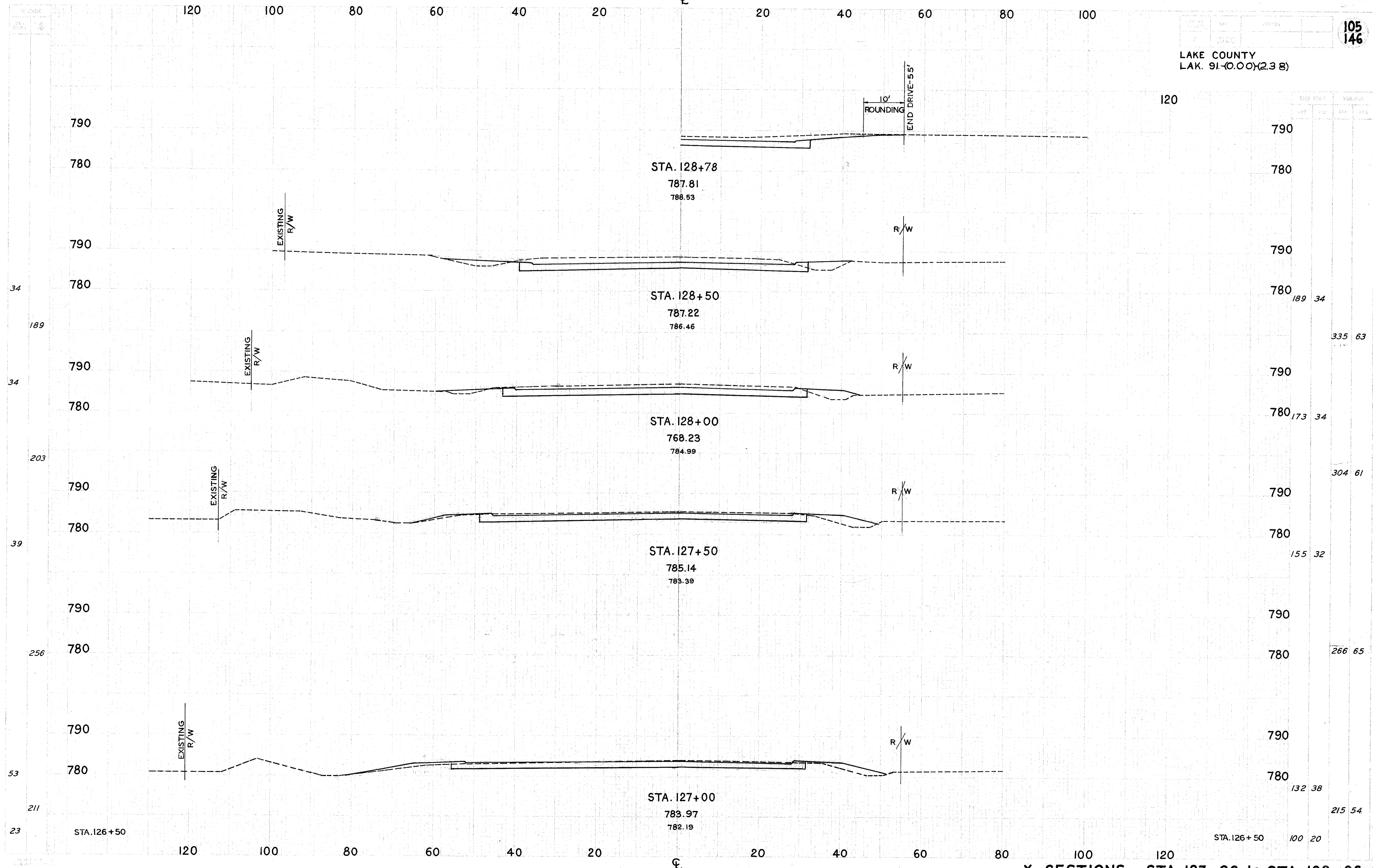
X-SECTIONS ... STA. 127+00 to STA. 128+86
