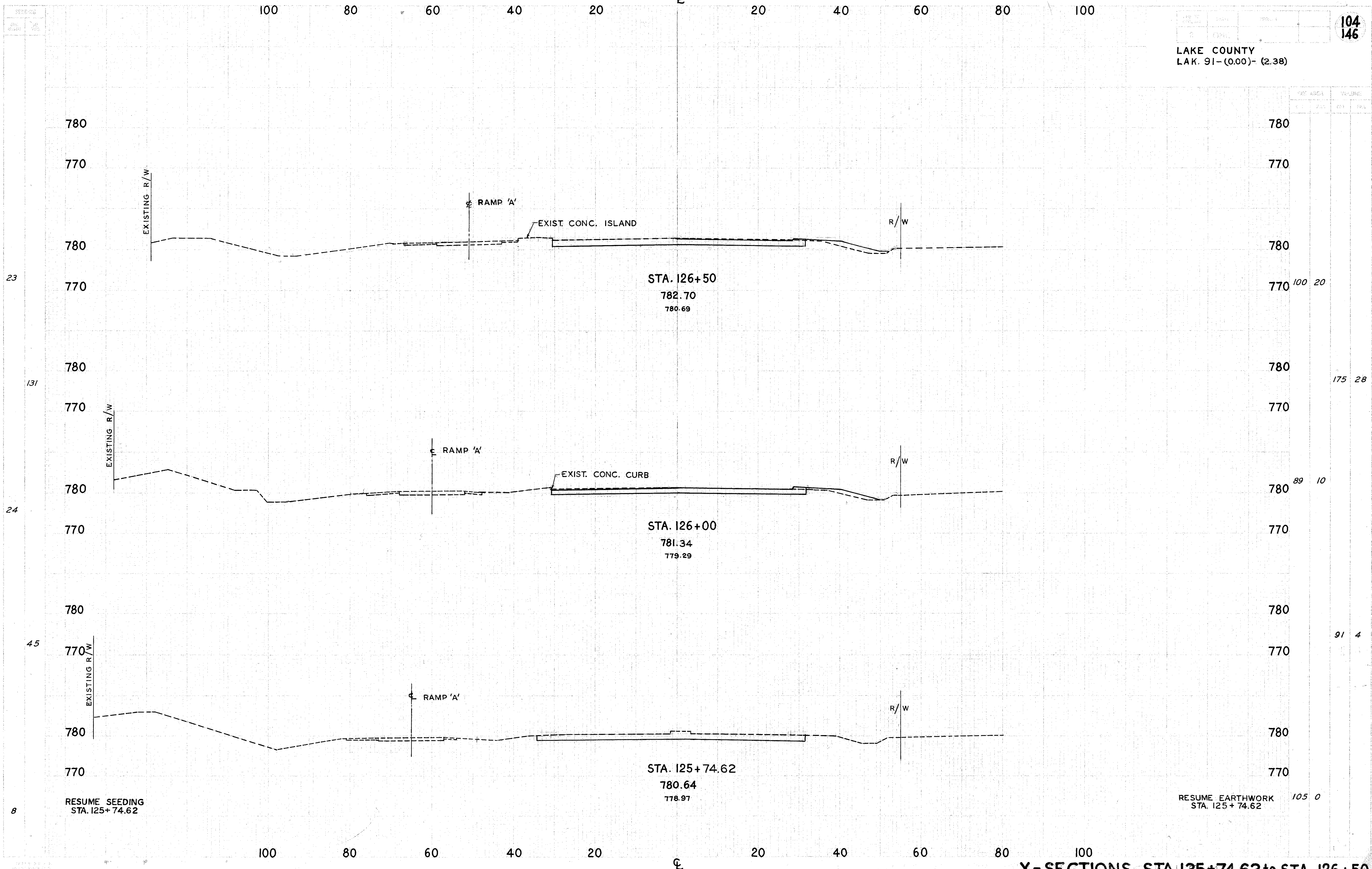
X-SECTIONS STA. 125+74.62 to STA. 126+50
