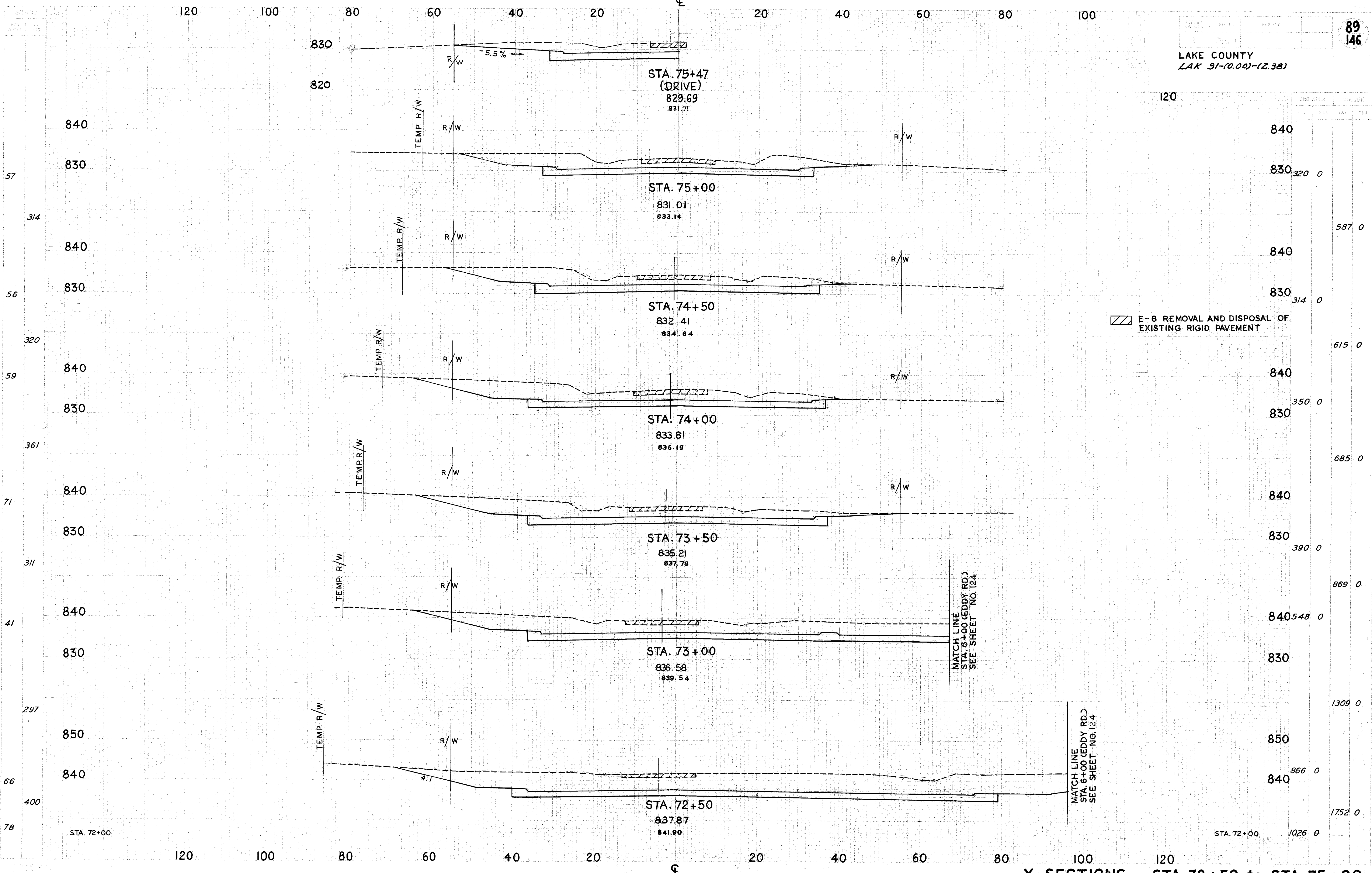
X-SECTIONS ... STA. 72+50 to STA. 75+00
