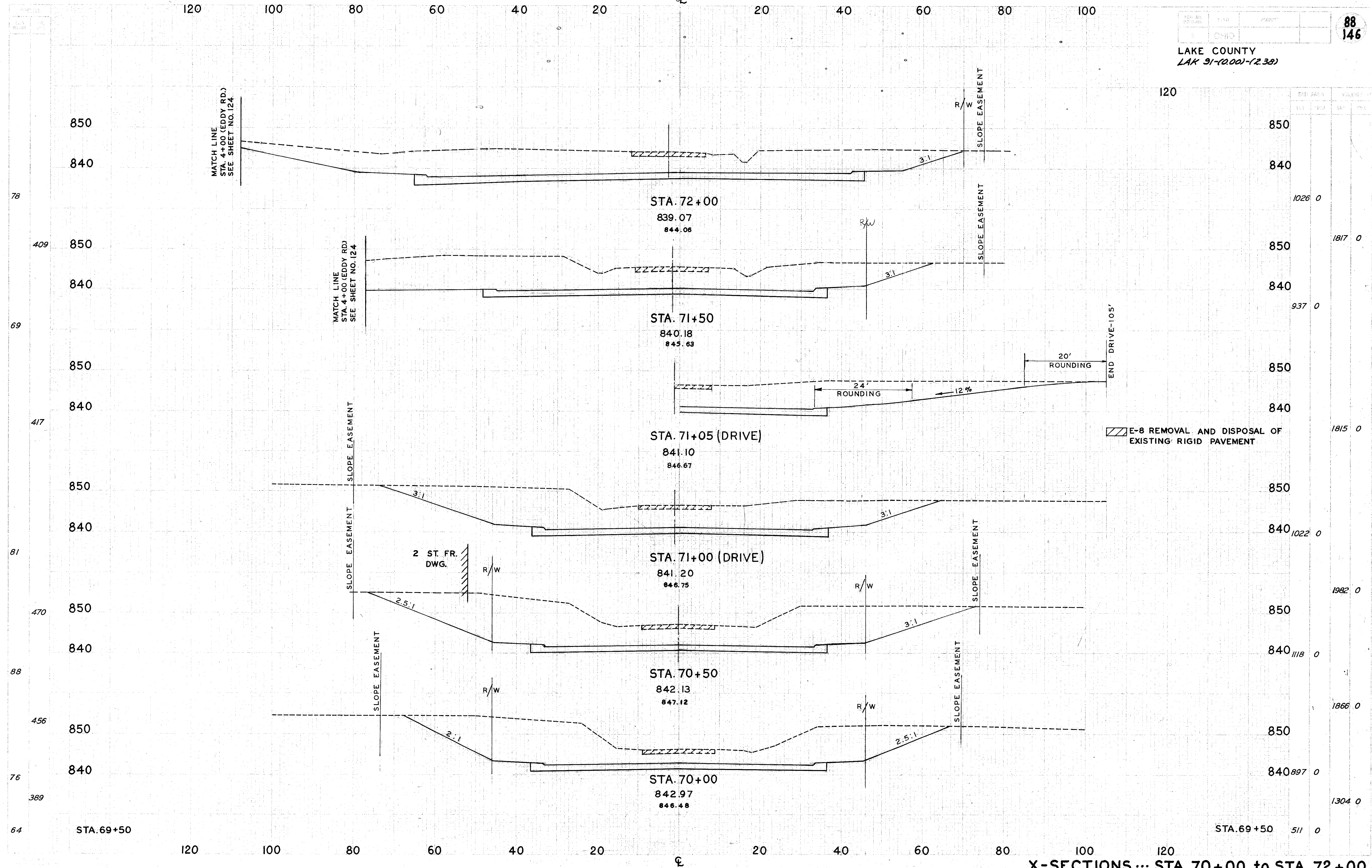
X-SECTIONS ... STA. 70+00 to STA. 72+00
