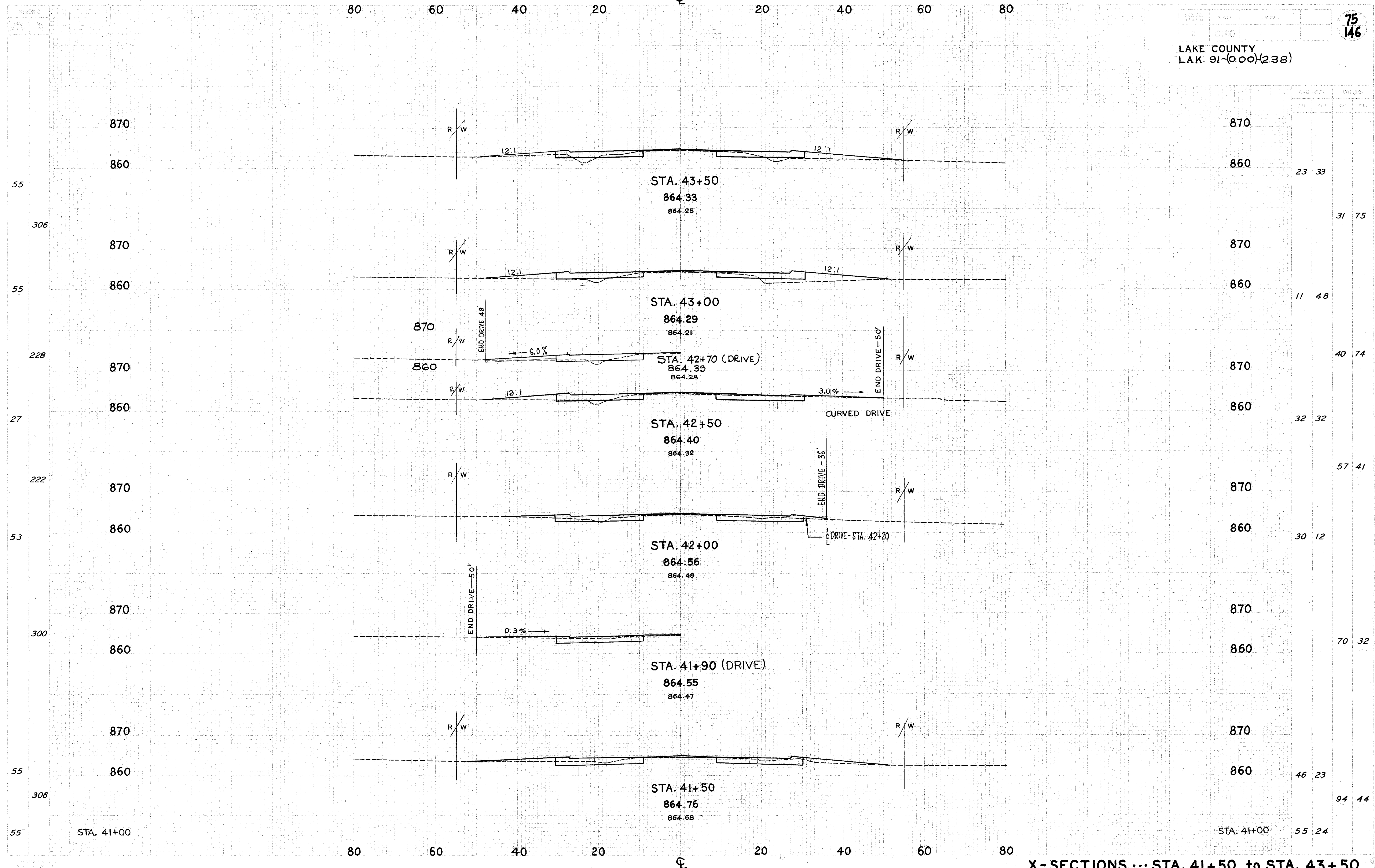
X-SECTIONS ... STA. 41+50 to STA. 43+50
