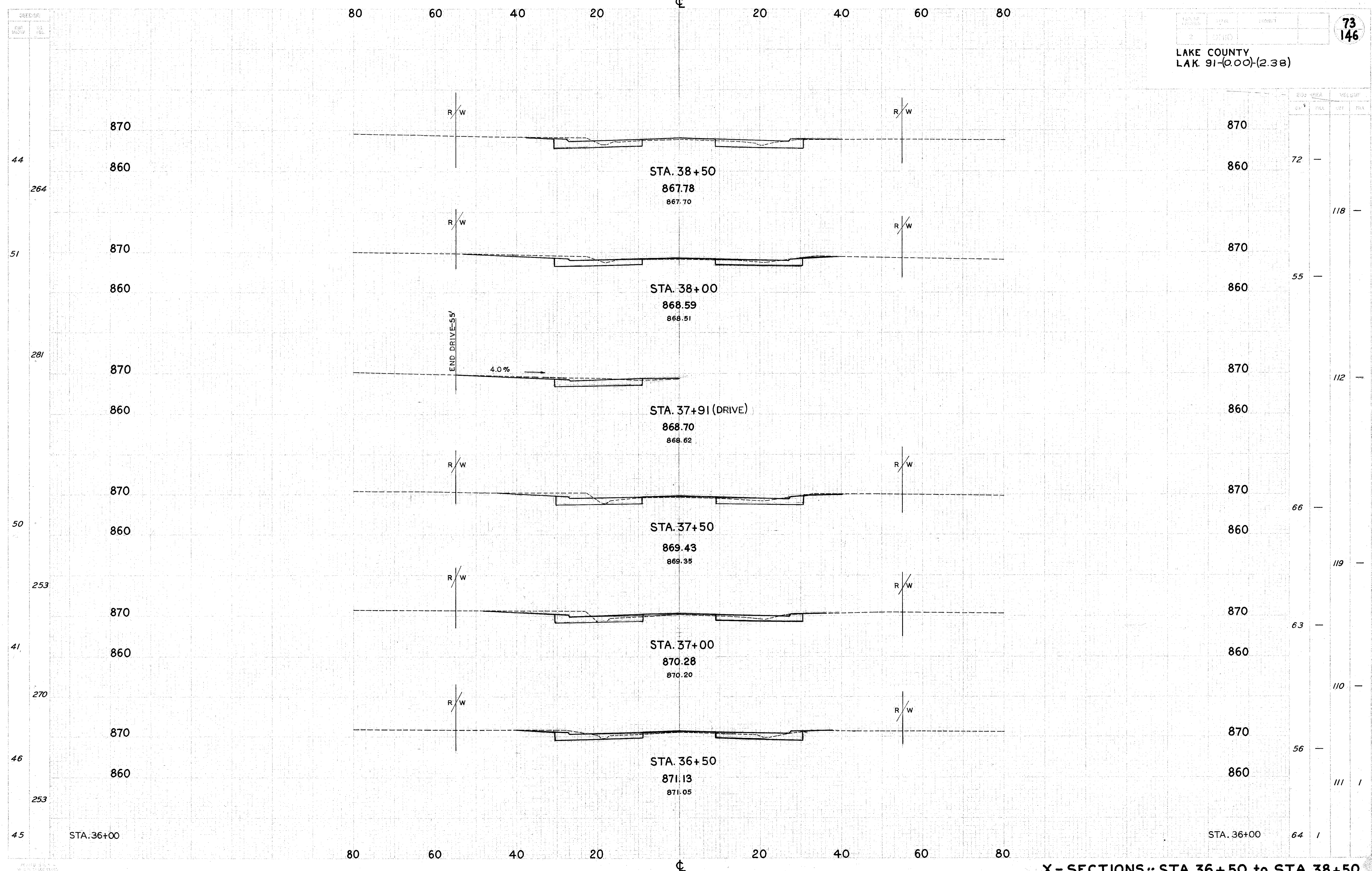
X-SECTIONS - STA. 36+50 to STA. 38+50
