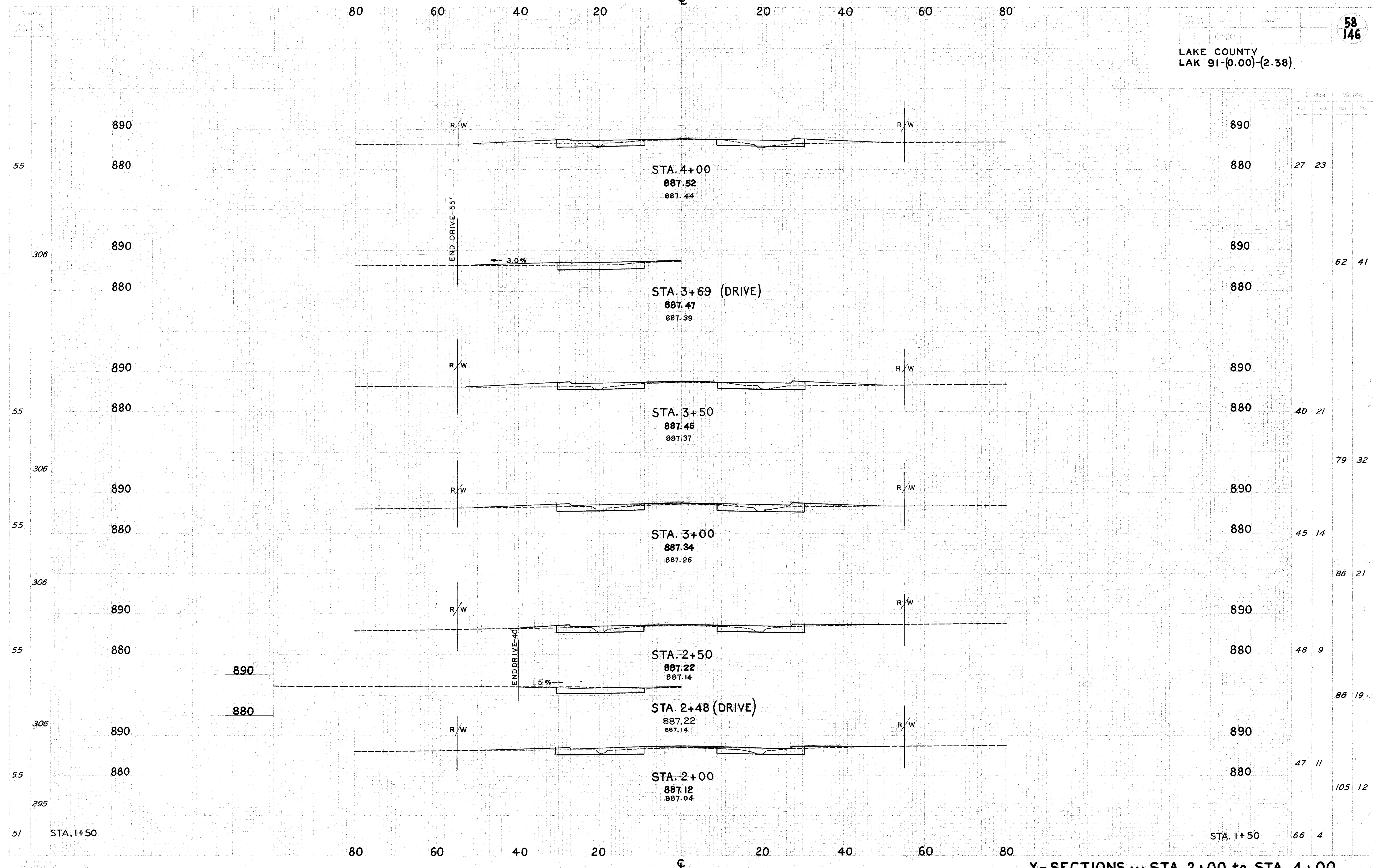
X-SECTIONS ... STA. 2+00 to STA. 4+00
