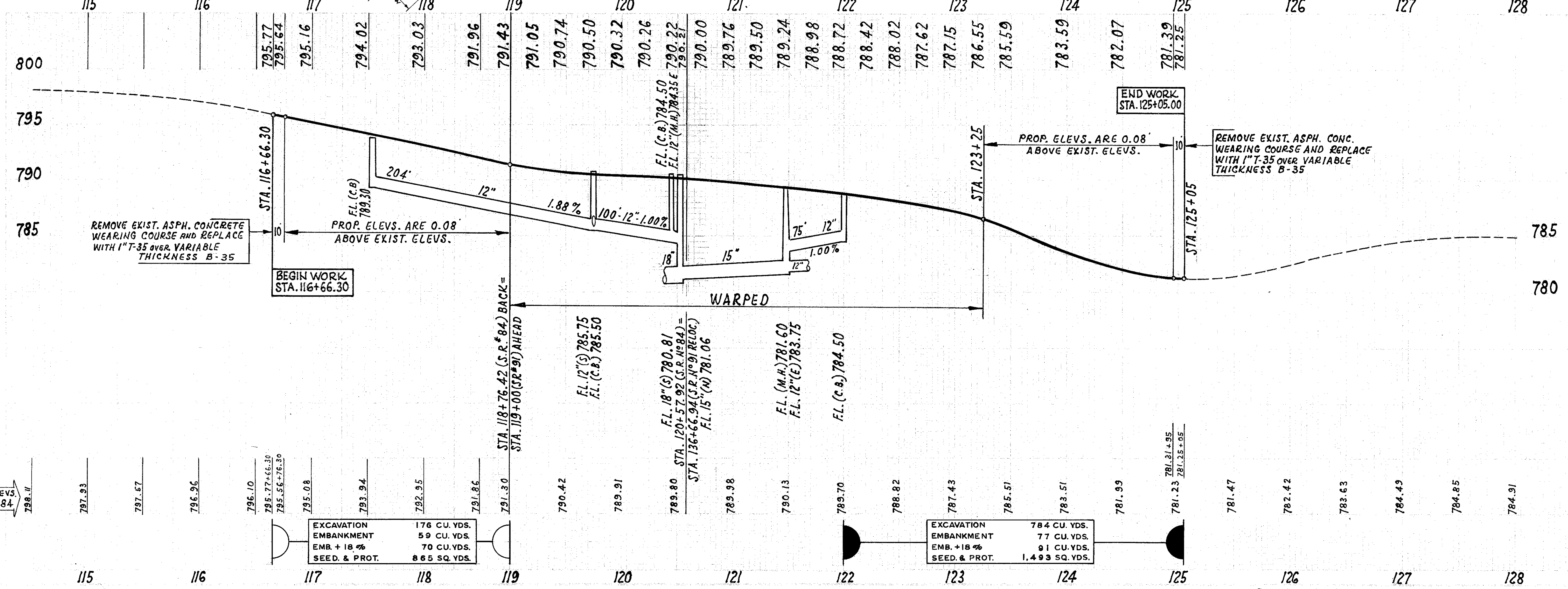
PLAN & PROFILE - S.R. No 84 - STA. 115+00 to STA. 128+00
