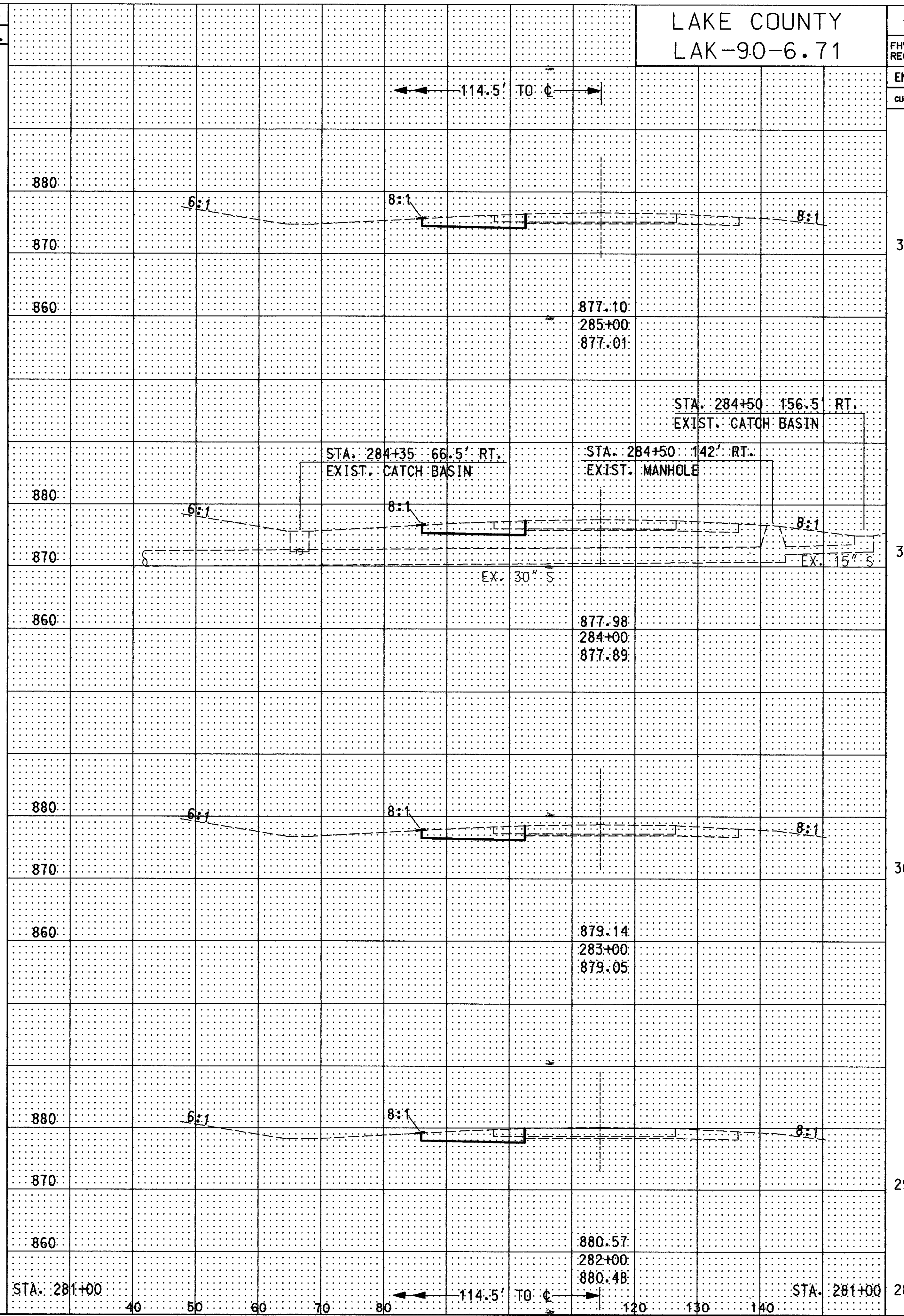
CROSS SECTION STA. 282+00 TO STA. 285+00 (WB) STA. 282+00 TO STA. 285+00 (EB)
