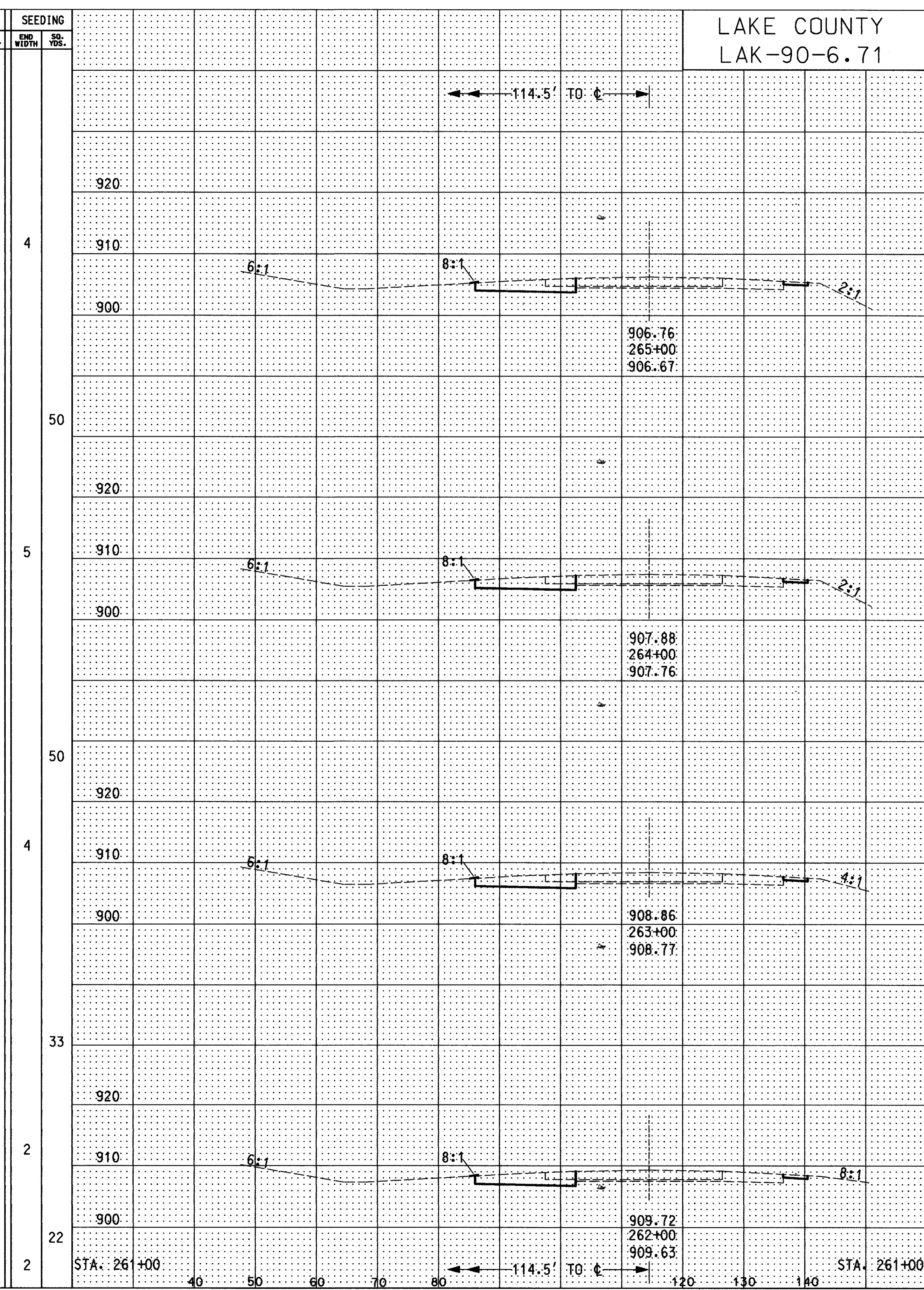
CROSS SECTION STA. 262+00 TO STA. 265+00 (WB) STA. 262+00 TO STA. 265+00 (EB)
