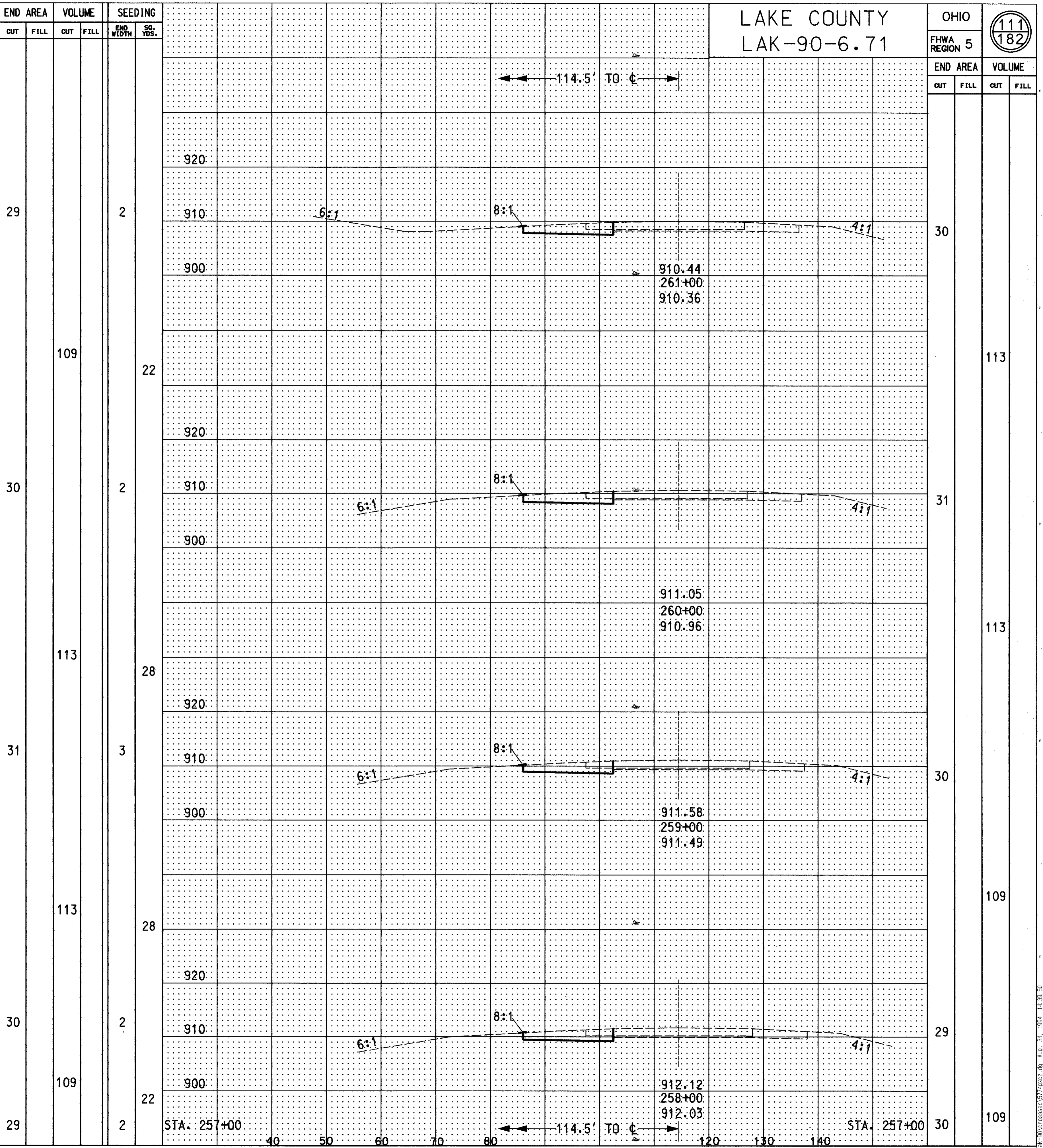
CROSS SECTION STA. 258+00 TO STA. 261+00 (WB) STA. 258+00 TO STA. 261+00 (EB)
