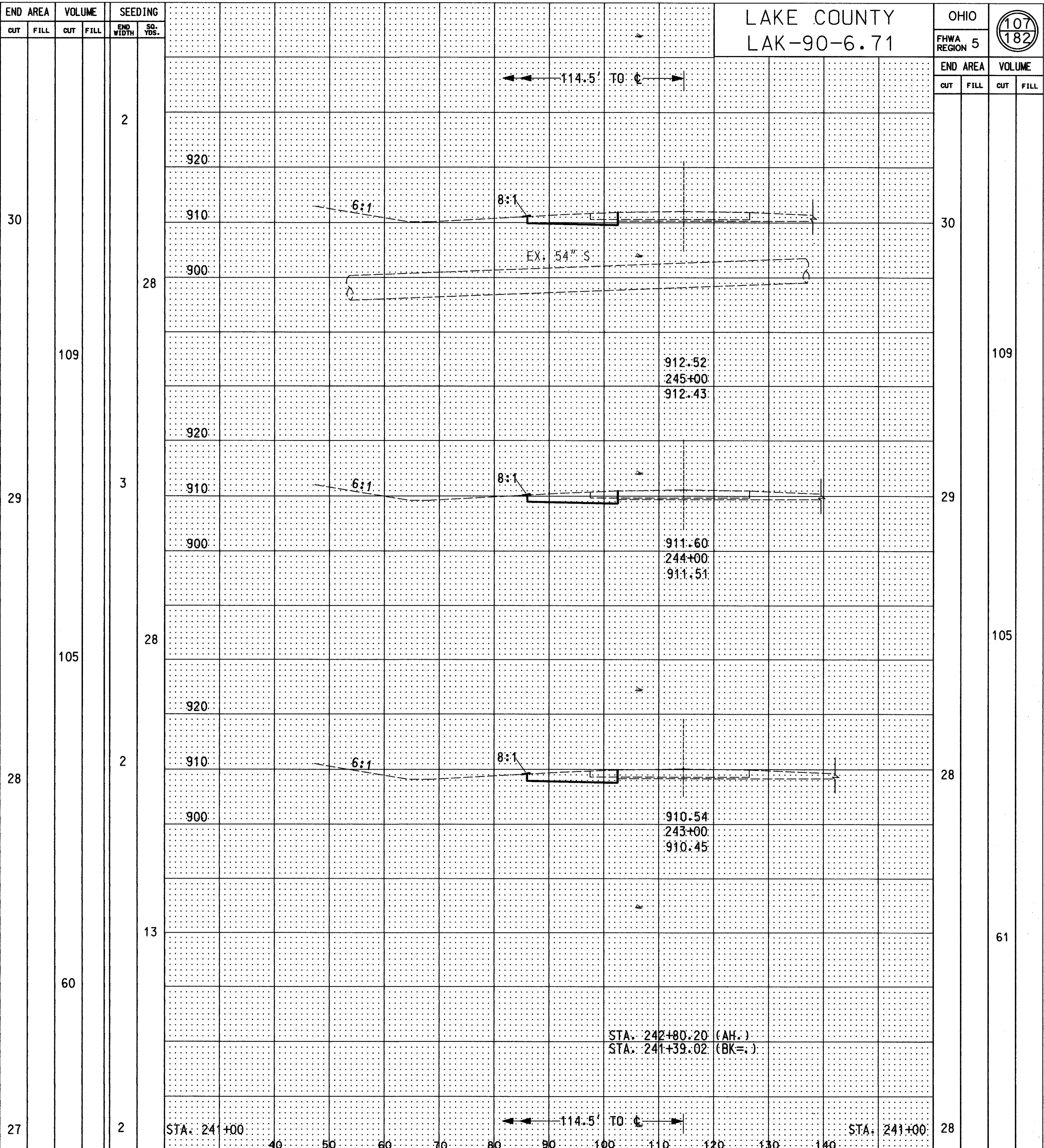
CROSS SECTION STA. 242+00 TO STA. 245+00 (WB) STA. 242+00 TO STA. 245+00 (EB)
