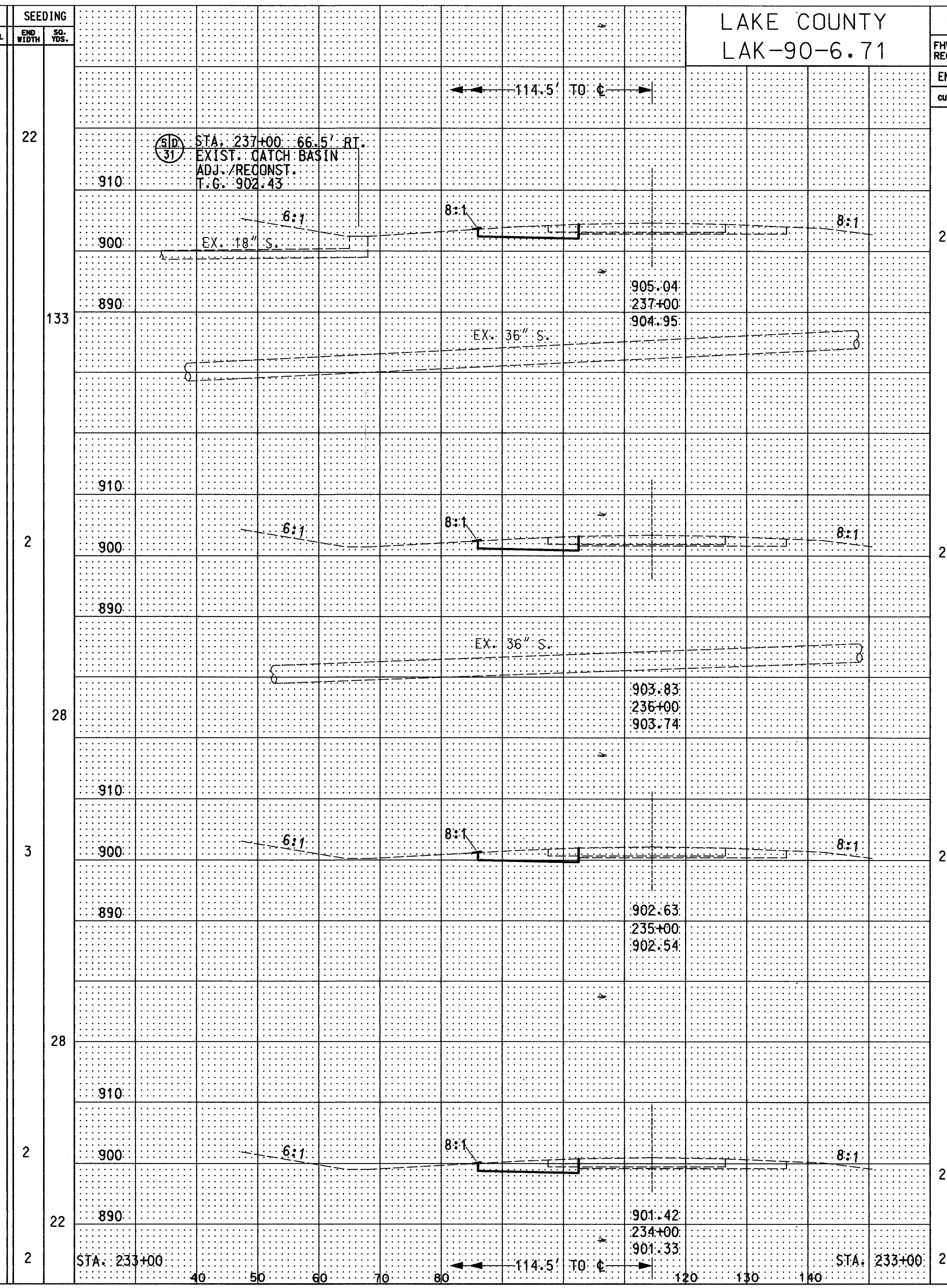
CROSS SECTION STA. 234+00 TO STA. 237+00 (WB) STA. 234+00 TO STA. 237+00 (EB)
