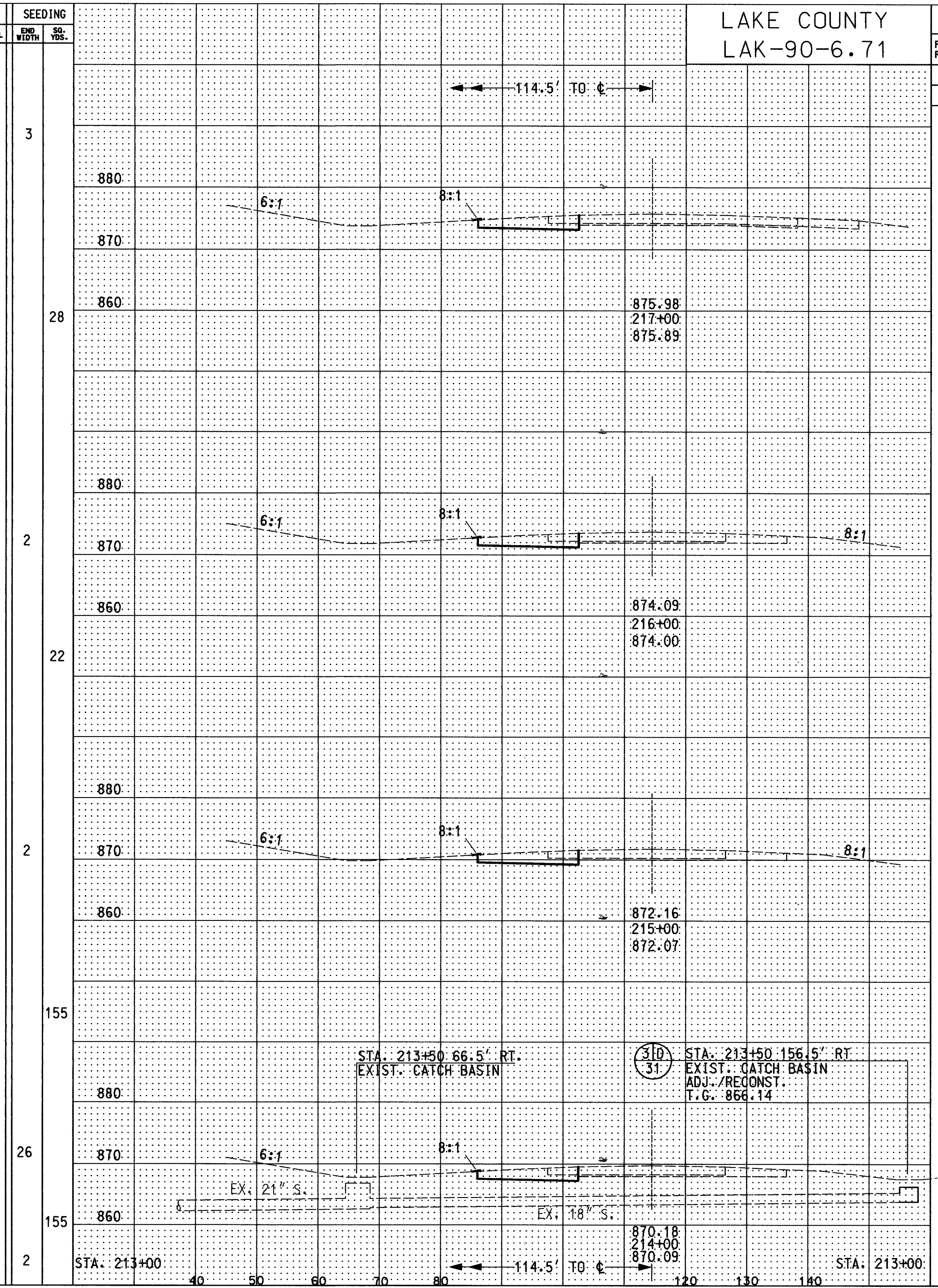
CROSS SECTION STA. 214+00 TO STA. 217+00 (WB) STA. 214+00 TO 217+00 (EB)
