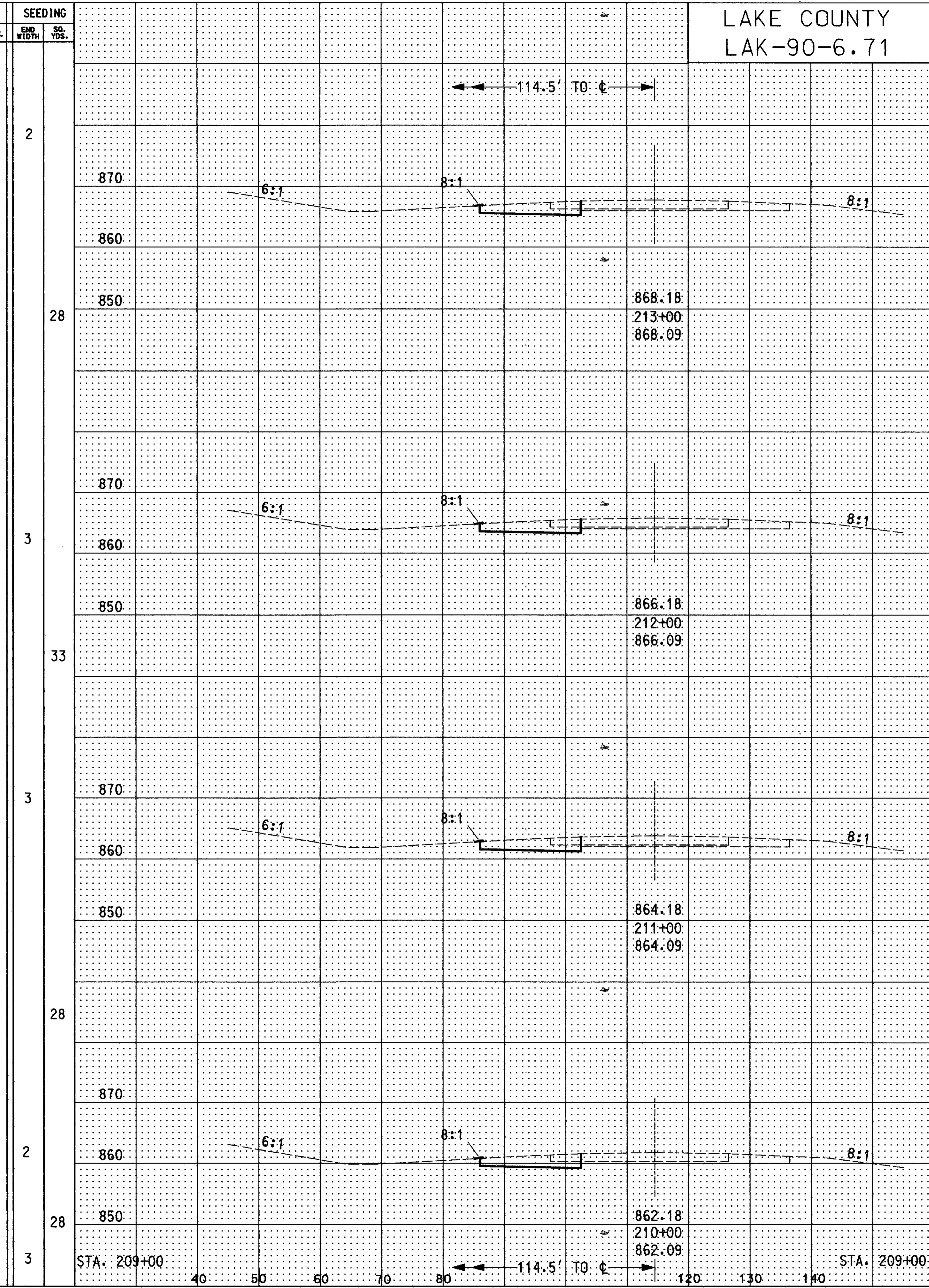
CROSS SECTION STA. 210+00 TO STA. 213+00 (WB) STA. 210+00 TO 213+00 (EB)
