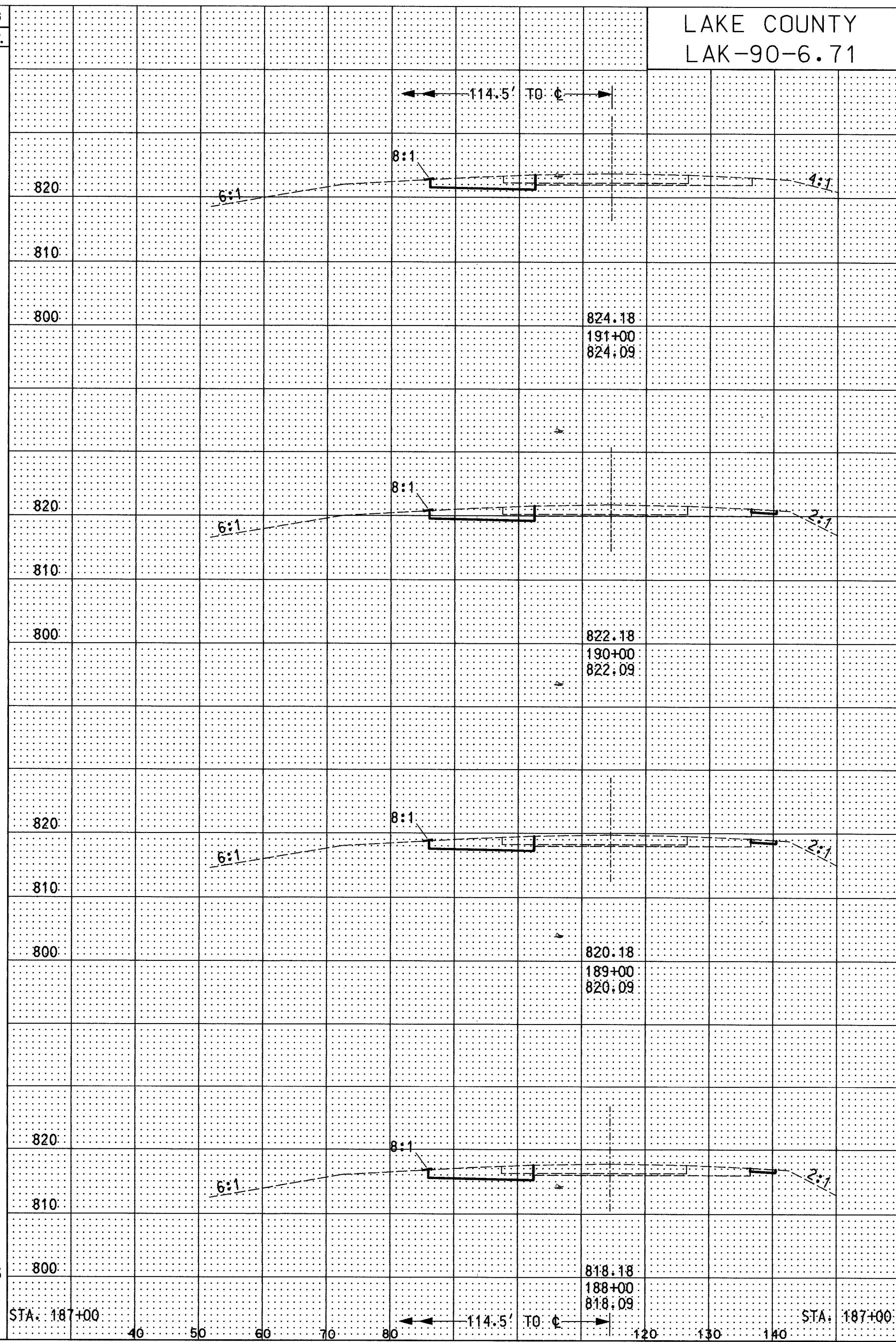
CROSS SECTION STA. 188+00 TO STA. 191+00 (WB) & STA. 188+00 TO STA. 191+00 (EB)
