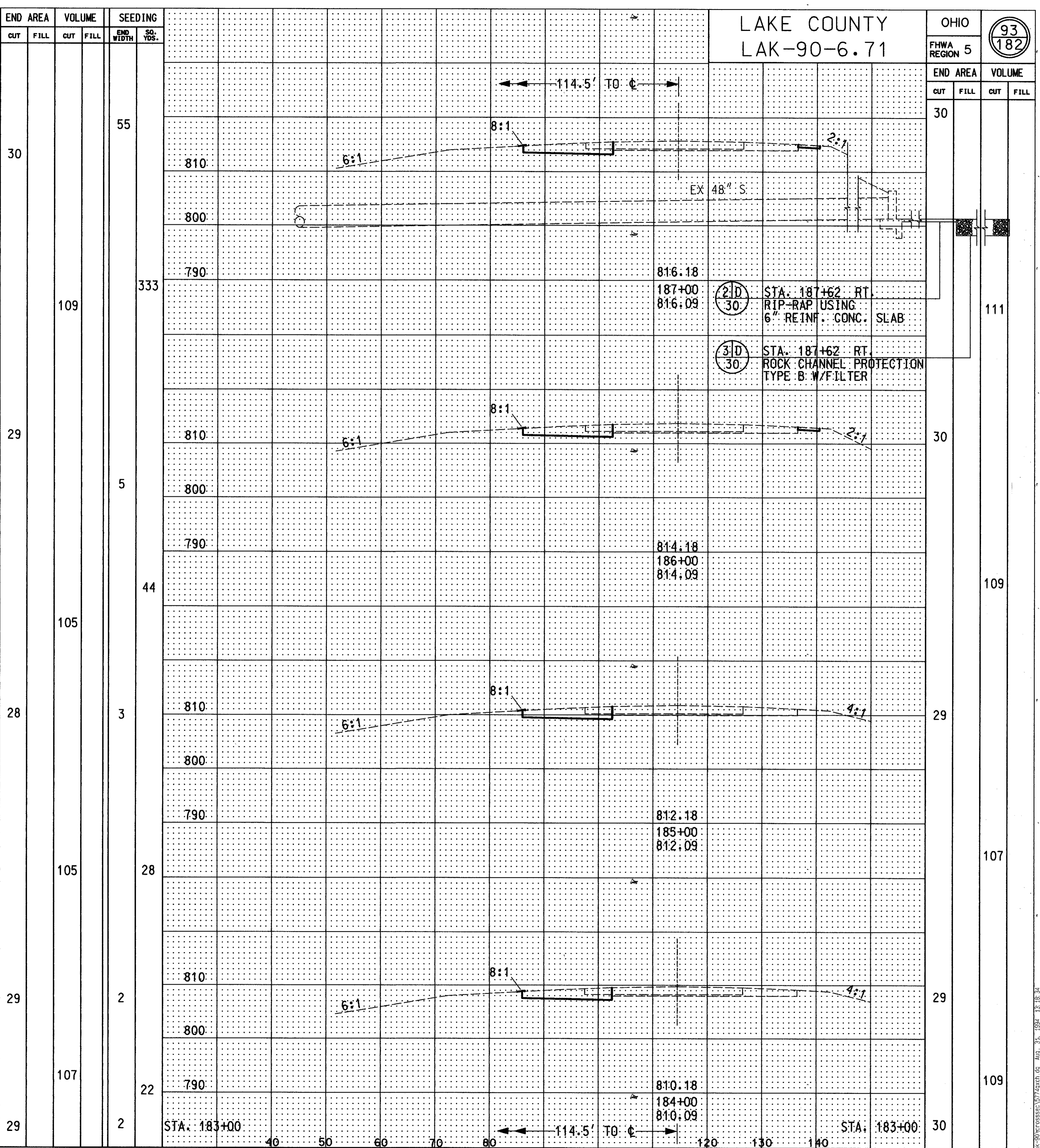
CROSS SECTION STA. 184+00 TO STA. 187+00 (WB) & STA. 184+00 TO STA. 187+00 (EB)
