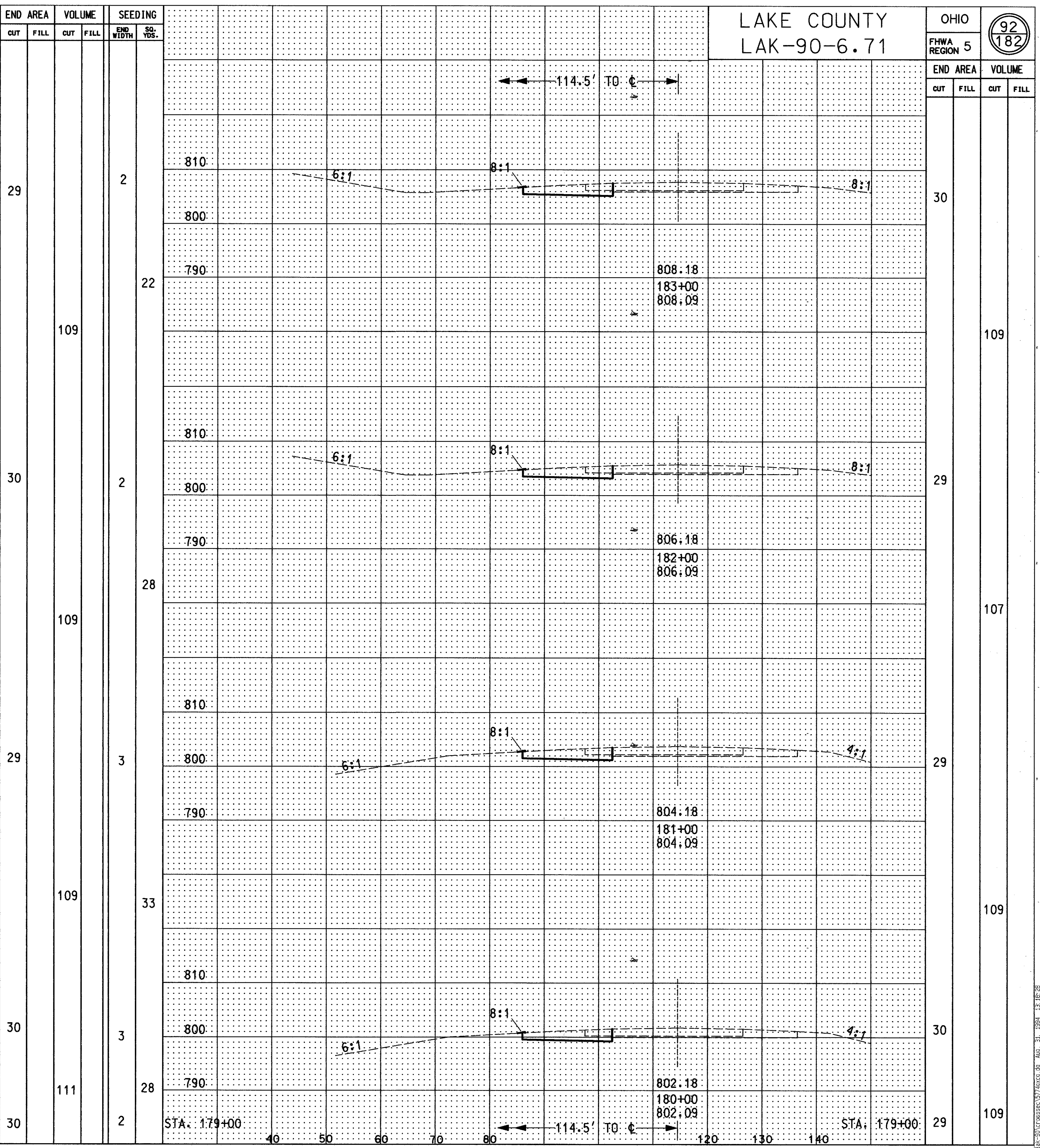
CROSS SECTION STA. 180+00 TO STA. 183+00 (WB) & STA. 180+00 TO STA. 183+00 (EB)
