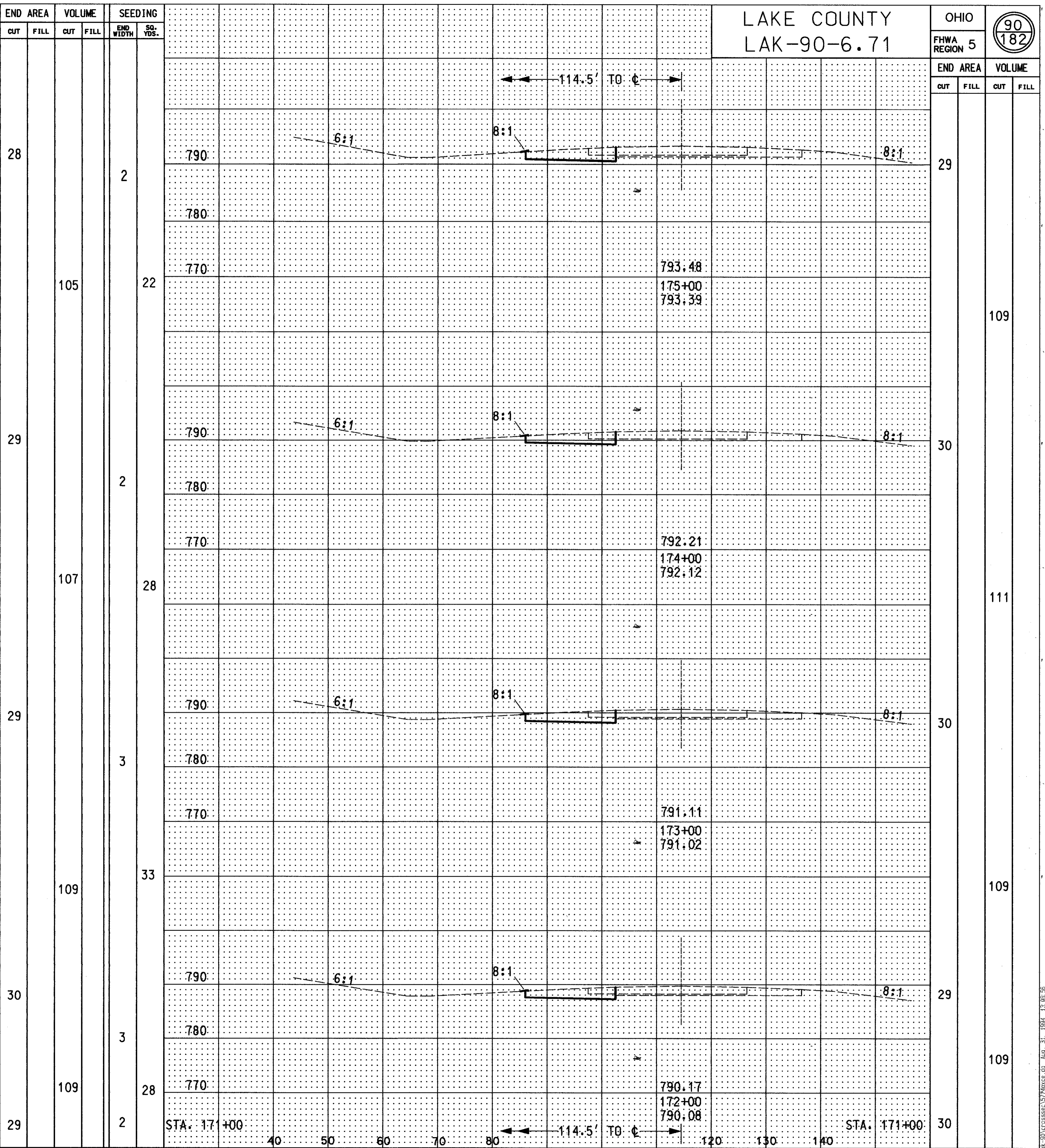
CROSS SECTION STA. 172+00 TO STA. 175+00 (WB) & STA. 172+00 TO 175+00 (EB)
