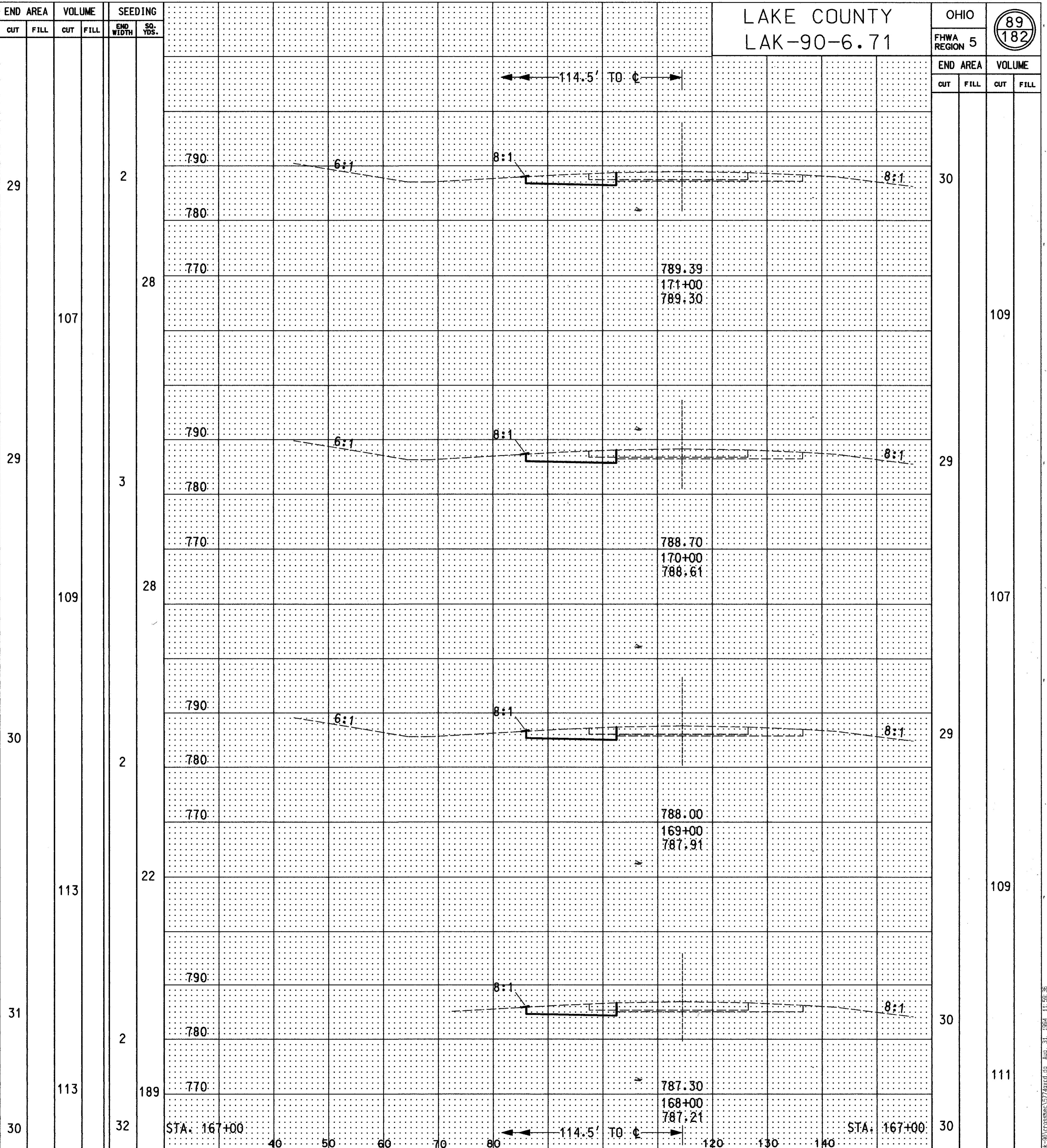
CROSS SECTION STA. 168+00 TO STA. 171+00 (WB) & STA. 168+00 TO STA. 171+00 (EB)
