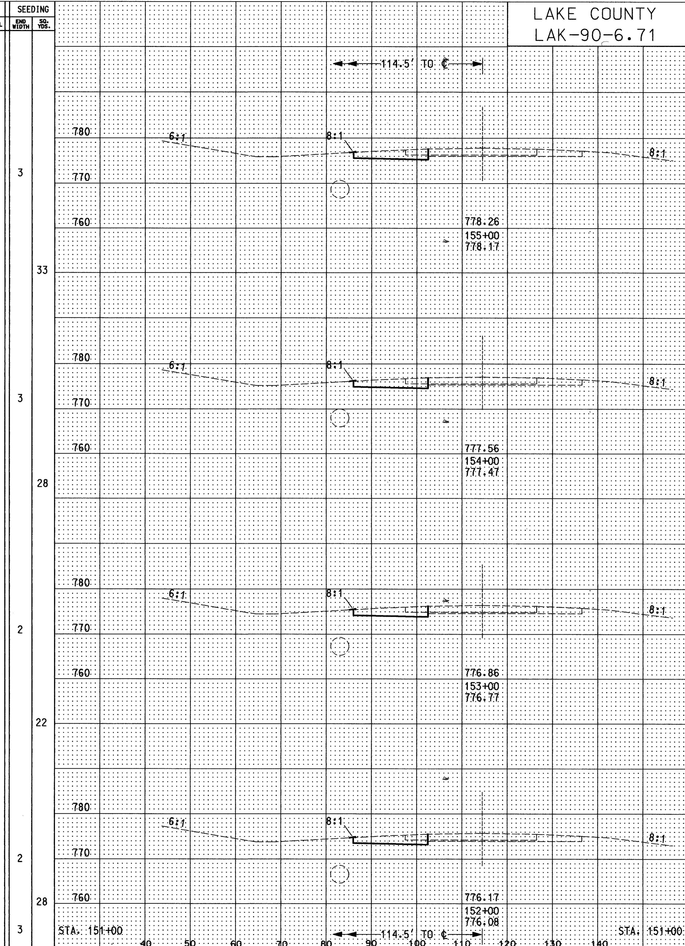
CROSS SECTION STA. 152+00 TO STA. 155+00 (WB) & STA. 152+00 TO STA. 155+00 (EB)
