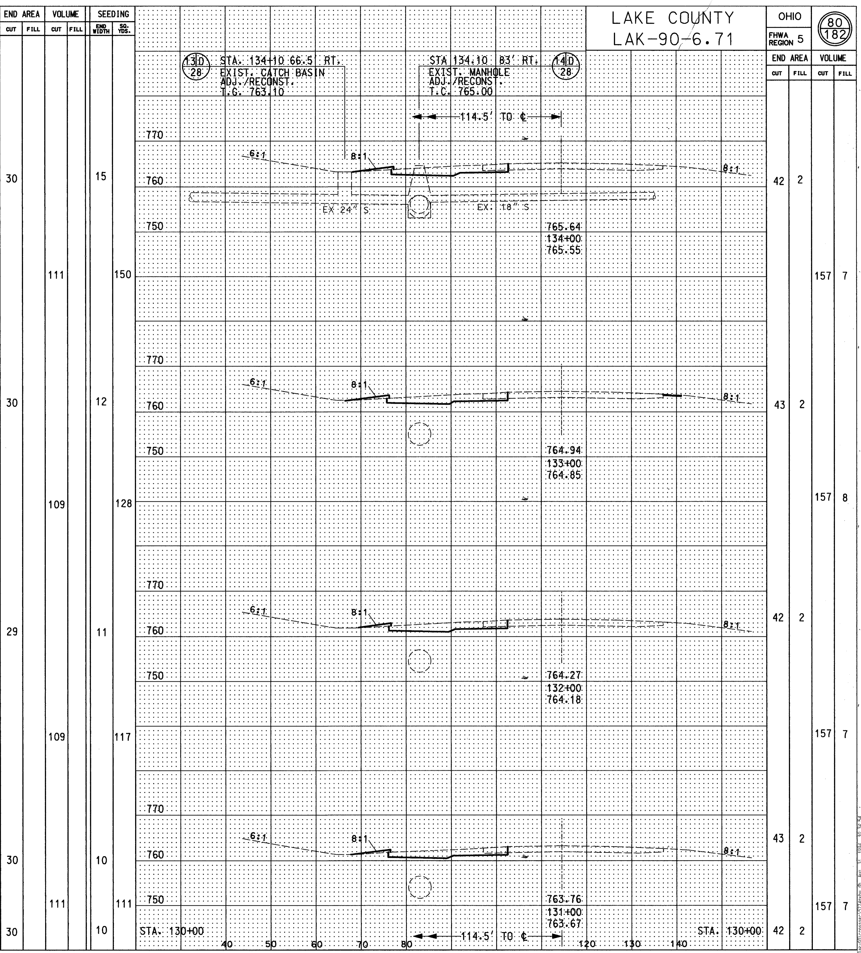
CROSS SECTION STA. 131+00 TO STA. 134+00 (WB) STA. 131+00 TO STA. 134+00 (EB)
