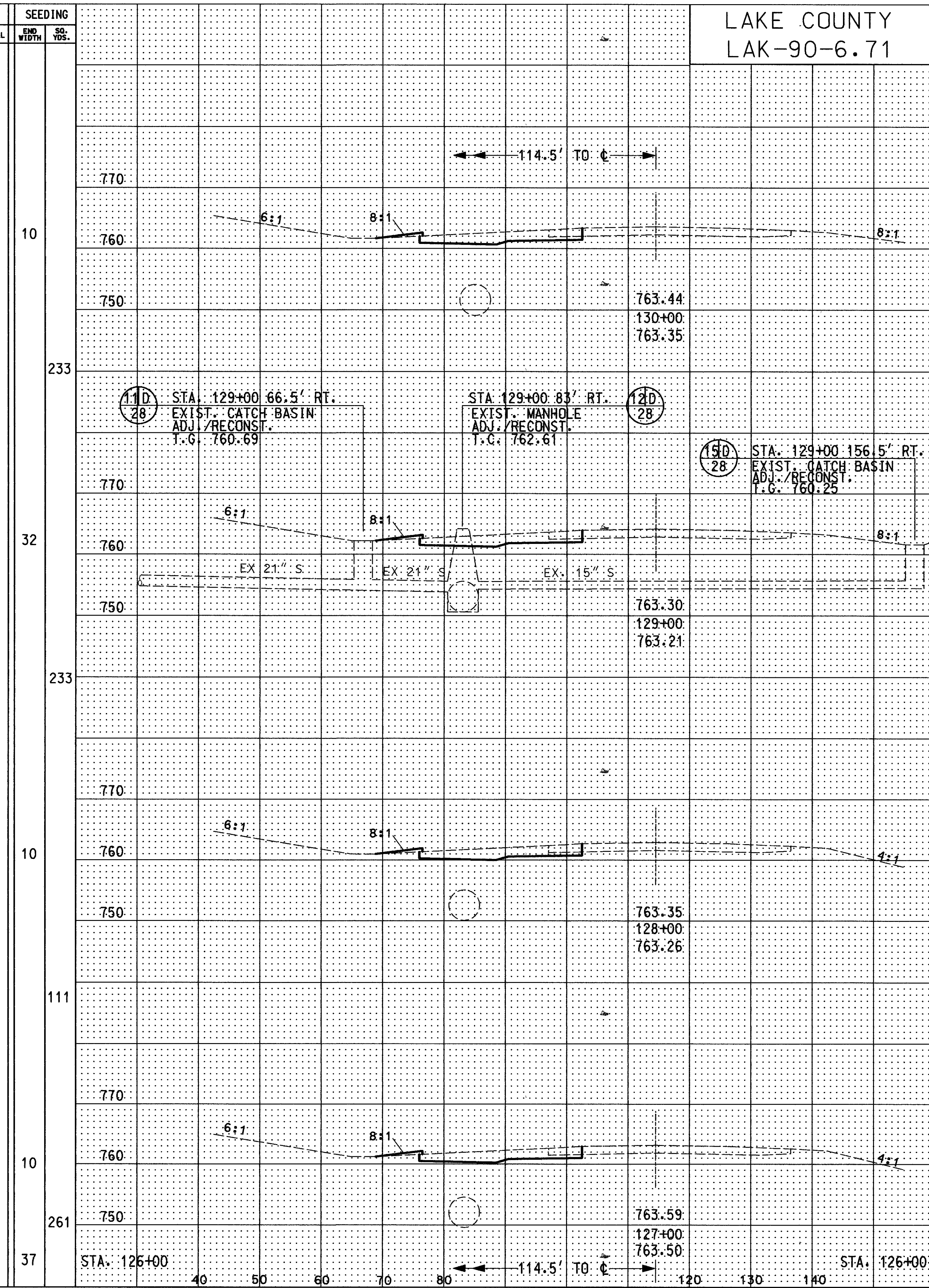
CROSS SECTION STA. 127+00 TO STA. 130+00 (WB) STA. 127+00 TO STA. 130+00 (EB)
