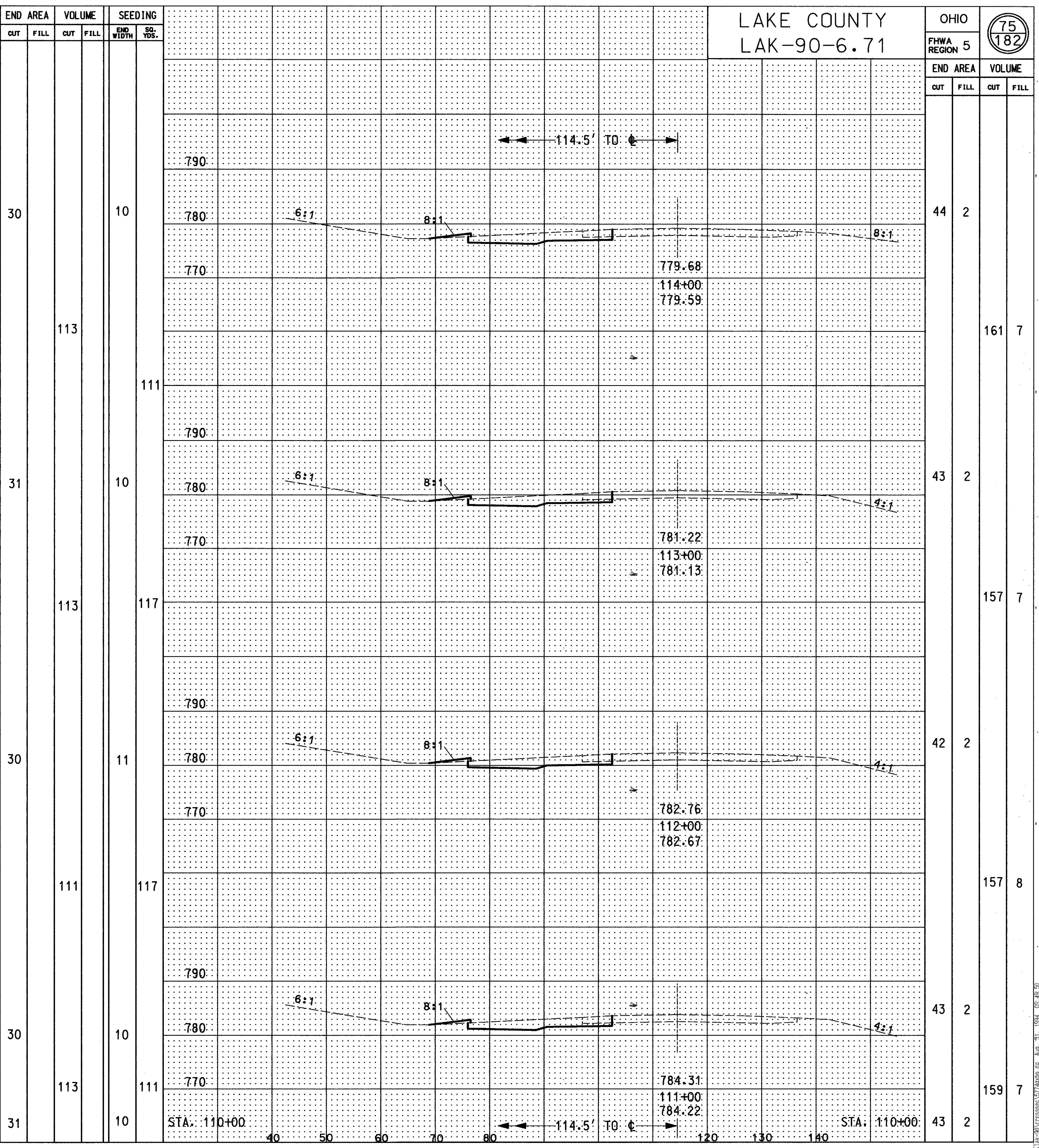
CROSS SECTION STA. 111+00 TO STA. 114+00 (WB) STA. 111+00 TO STA. 114+00 (EB)
