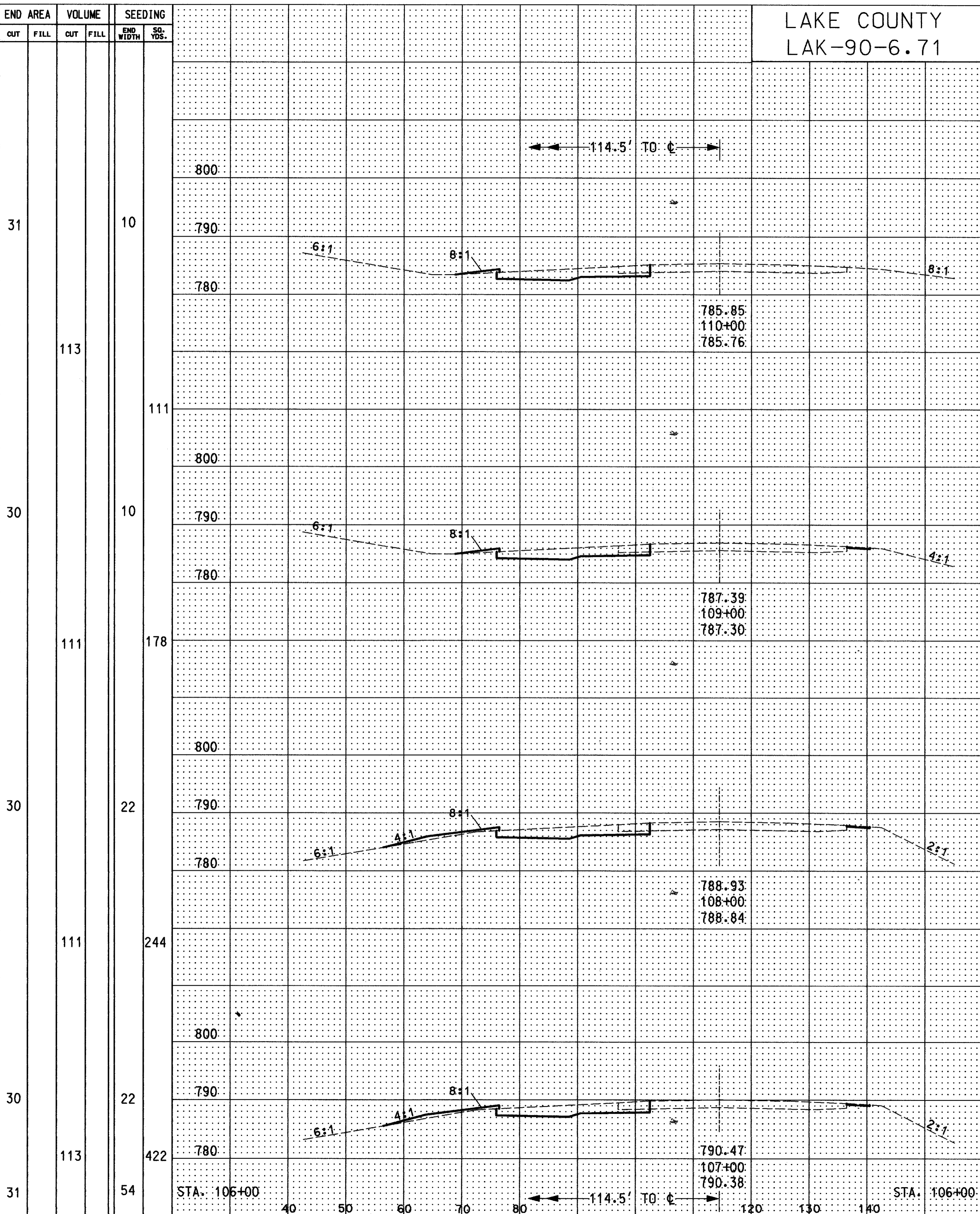
CROSS SECTION STA. 107+00 TO STA. 110+00 (WB) STA. 107+00 TO STA. 110+00 (EB)
