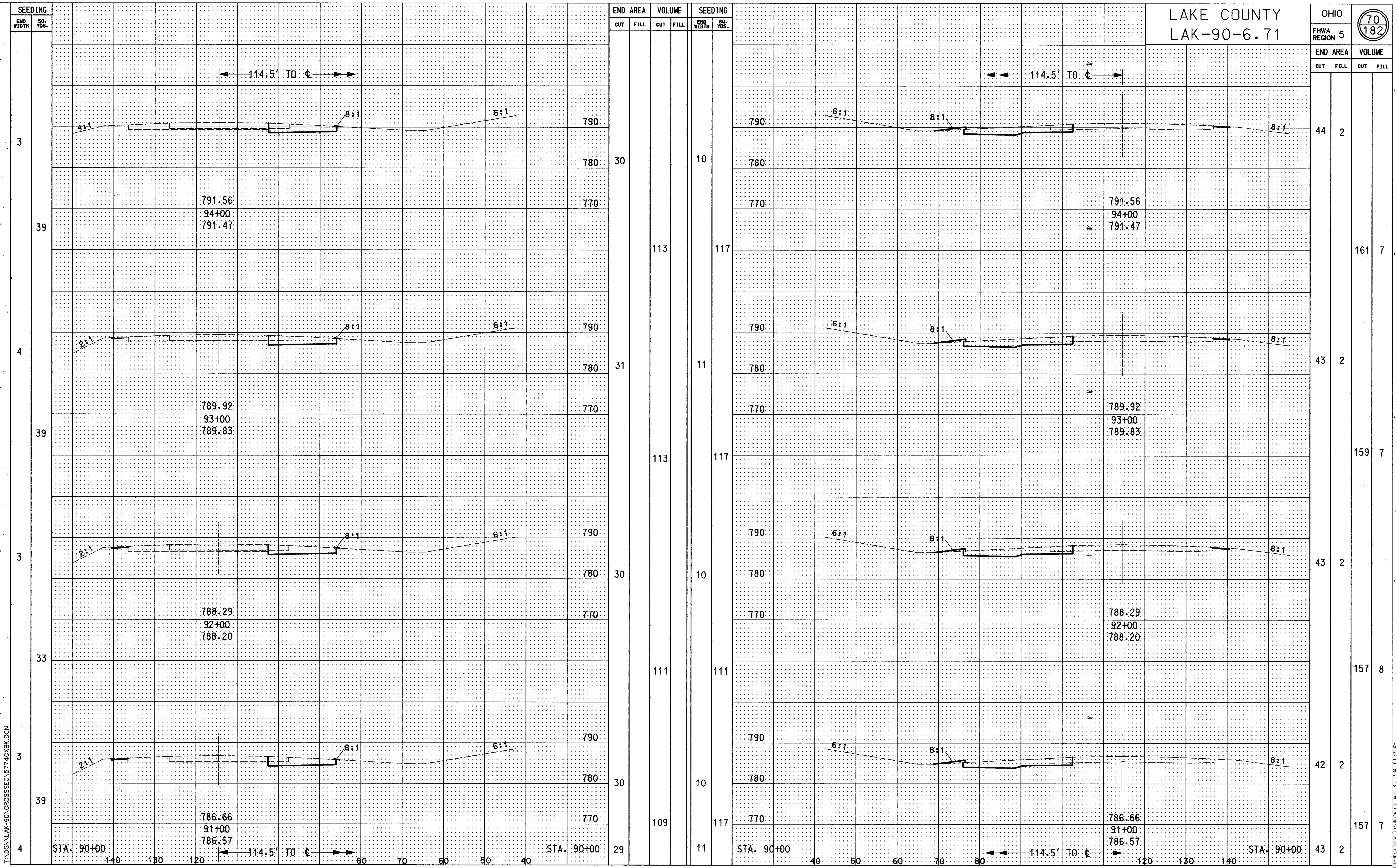
CROSS SECTION STA. 91+00 TO STA. 94+00 (WB) STA. 91+00 TO STA. 94+00 (EB)
