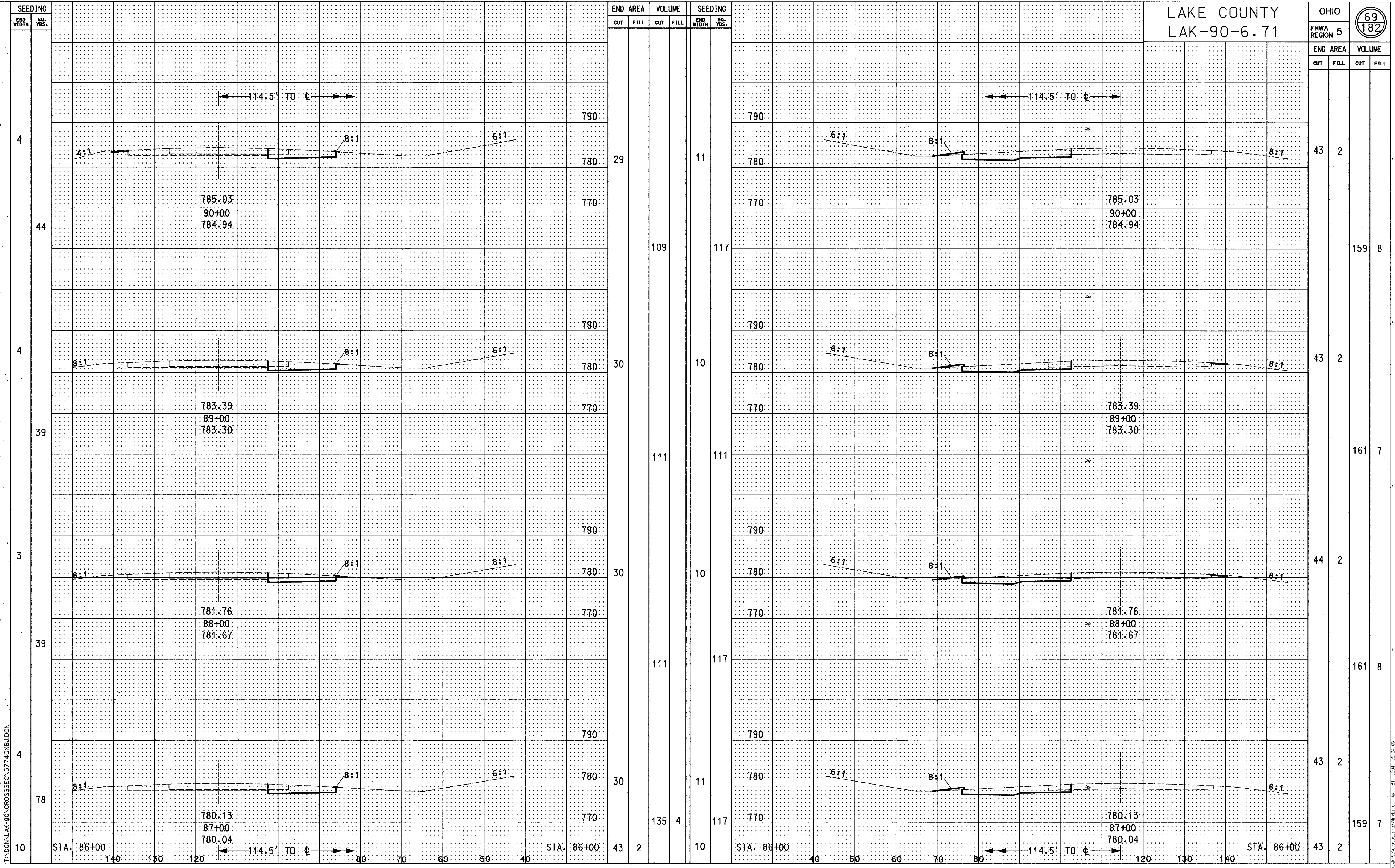
CROSS SECTION STA. 87+00 TO STA. 90+00 (WB) STA. 87+00 TO STA. 90+00 (EB)
