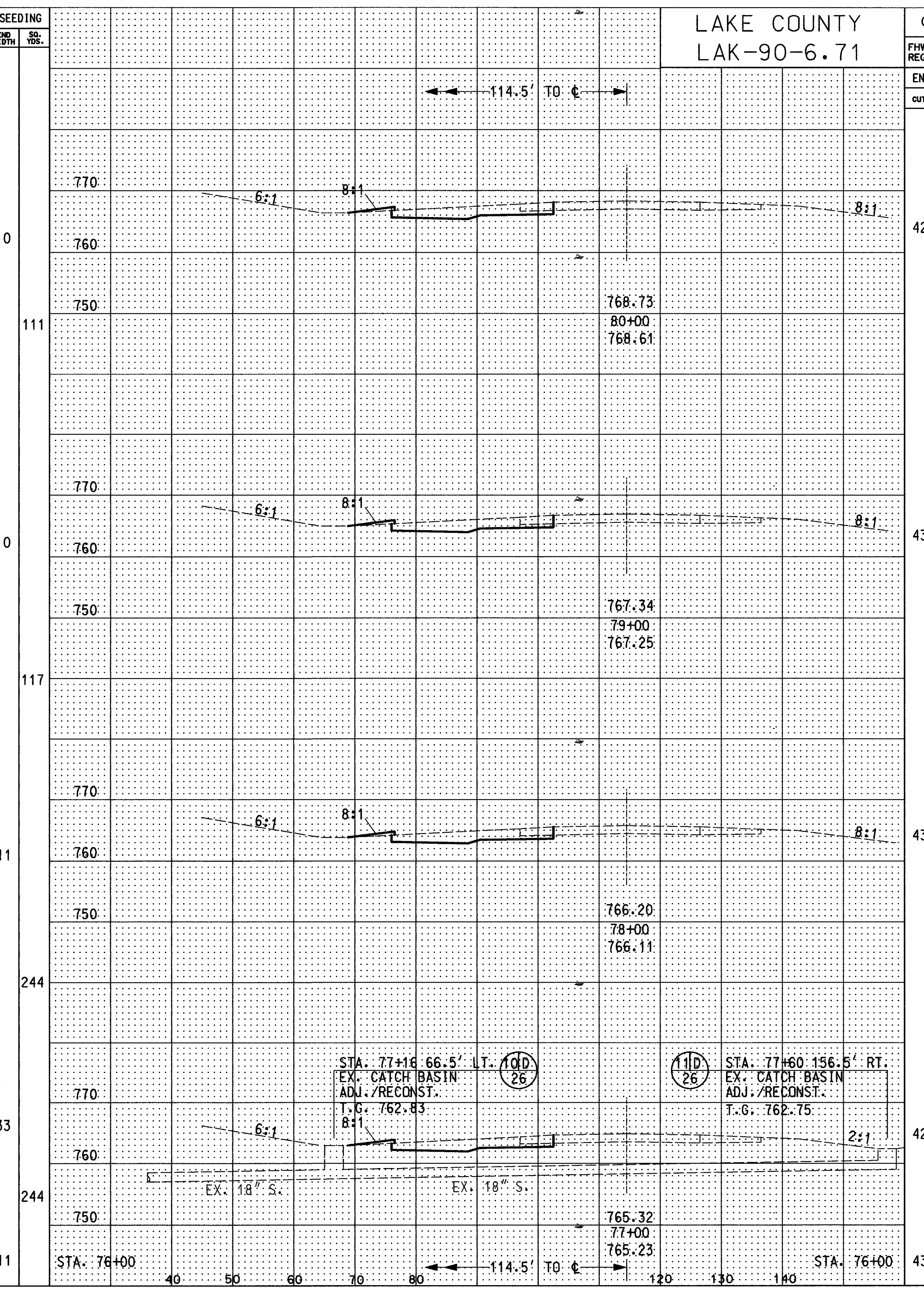
CROSS SECTION STA. 77+00 TO STA. 80+00 (WB) STA. 77+00 TO STA. 80+00 (EB)
