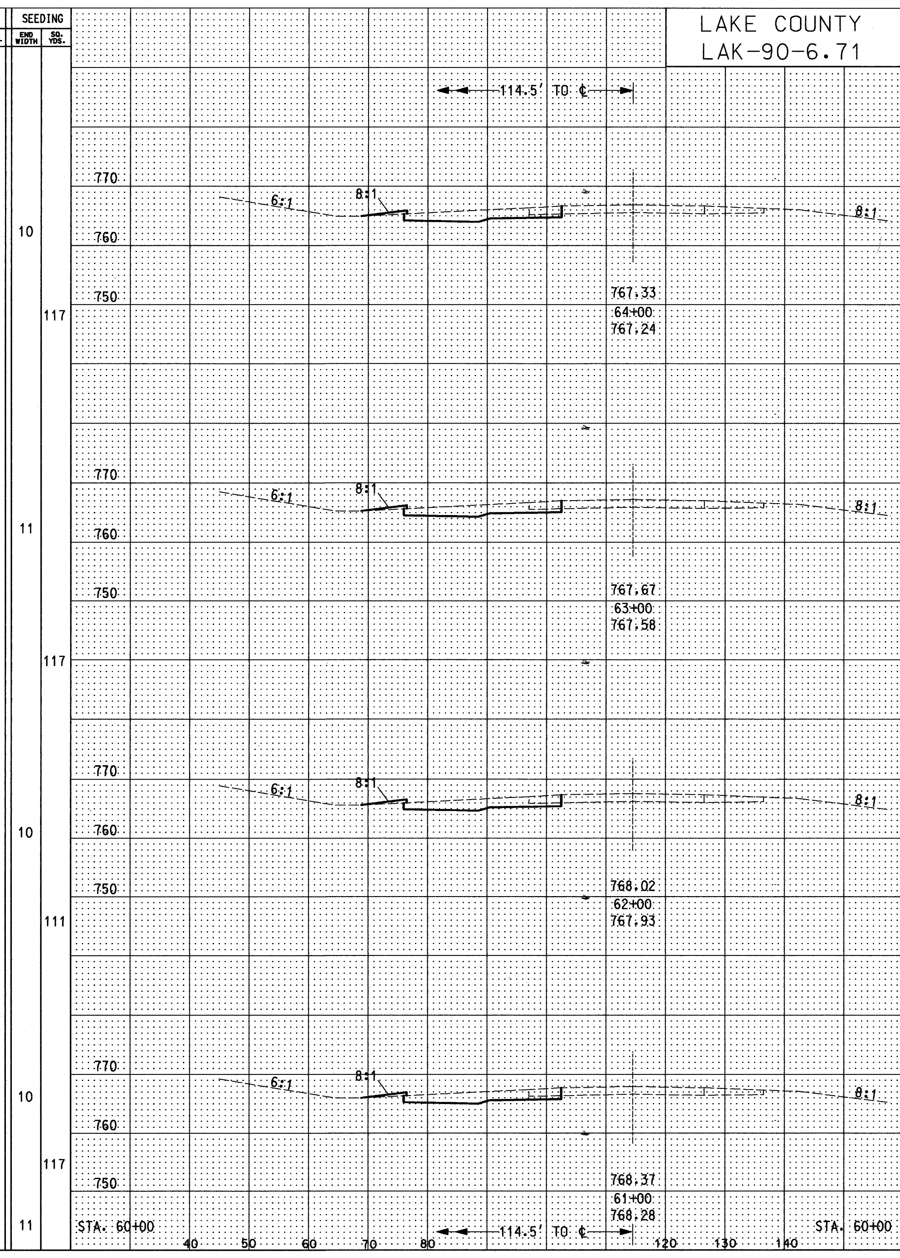
CROSS SECTION STA. 61+00 TO STA. 64+00 (WB) STA. 61+00 TO STA. 64+00 (EB)
