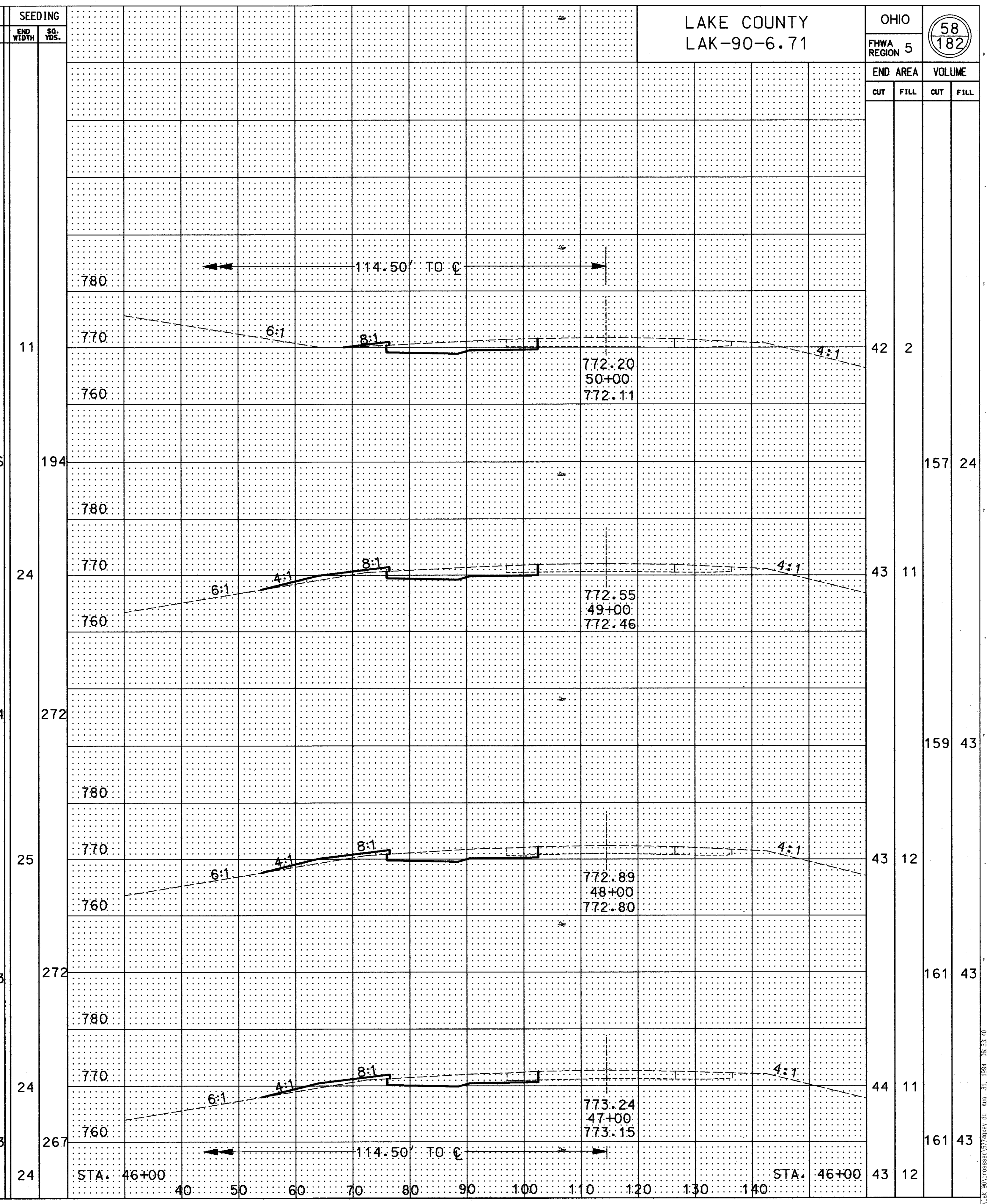
CROSS SECTIONS STA. 47+00 TO STA. 50+00 (WB) & STA. 47+00 TO STA. 50+00 (EB)
