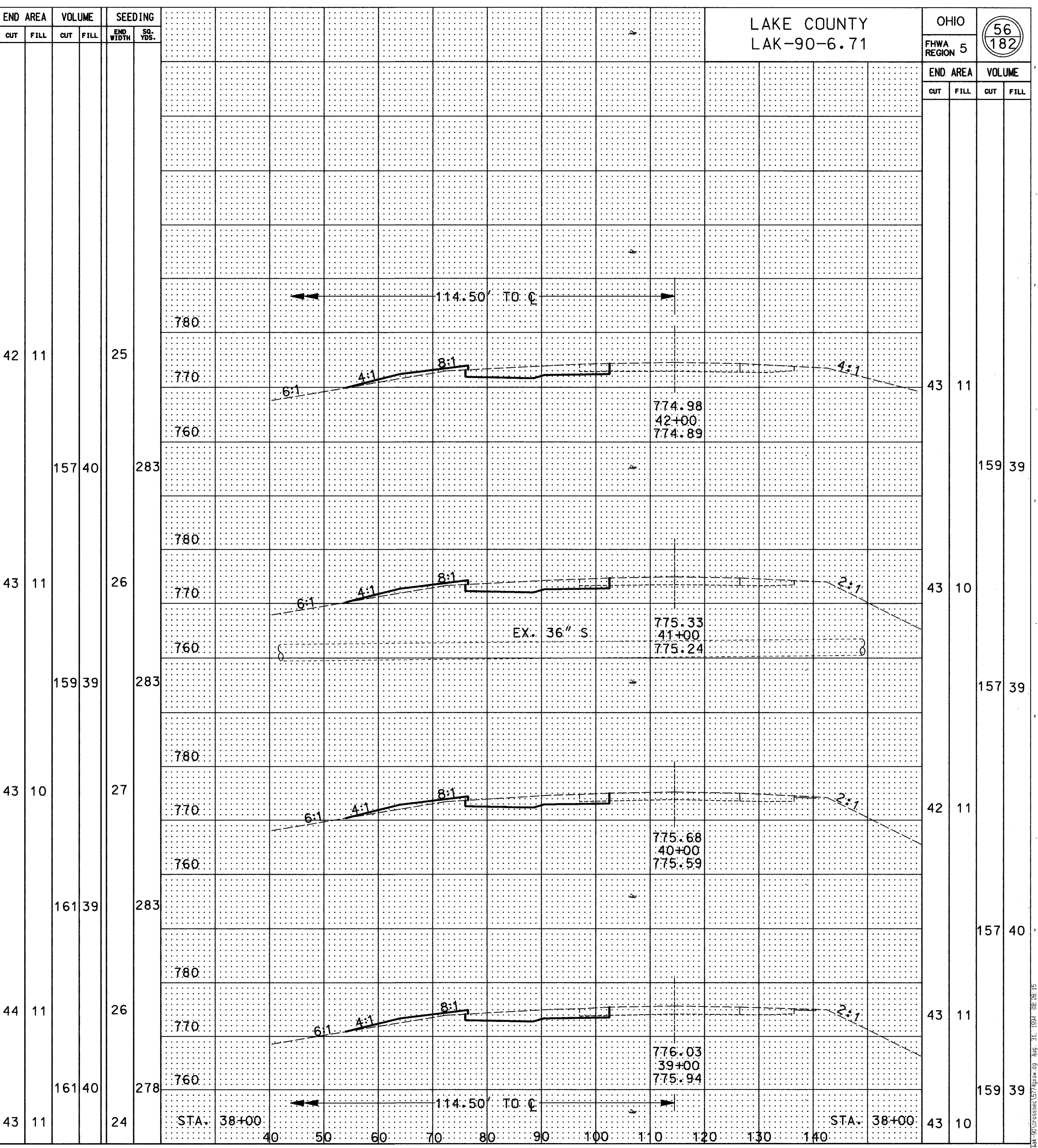
CROSS SECTIONS STA. 39+00 TO STA. 42+00 (WB) & STA. 39+00 TO STA. 42+00 (EB)
